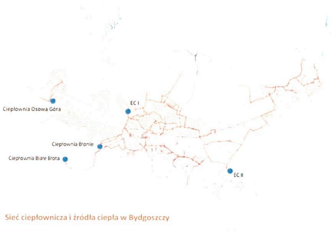
Rysunek 11. System zaopatrzenia w ciepło miasta Bydgoszcz
