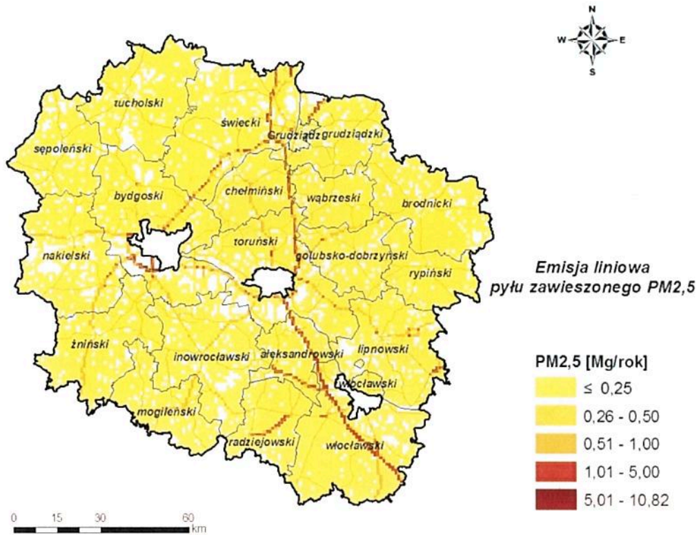
Rysunek 22. Emisja liniowa pyłu zawieszanego PM 2,5 z terenu strefy kujawsko-pomorskiej w 2015 r.
