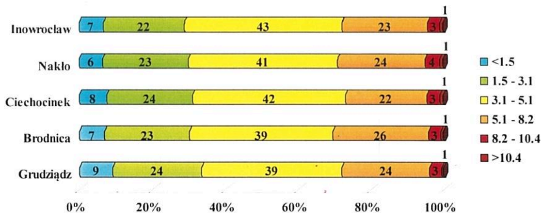
Rysunek 5. Procentowy rozkład prawdopodobieństwa występowania prędkości wiatru w określonych przedziałach, w strefie kujawsko-pomorskiej w 2015 r.
