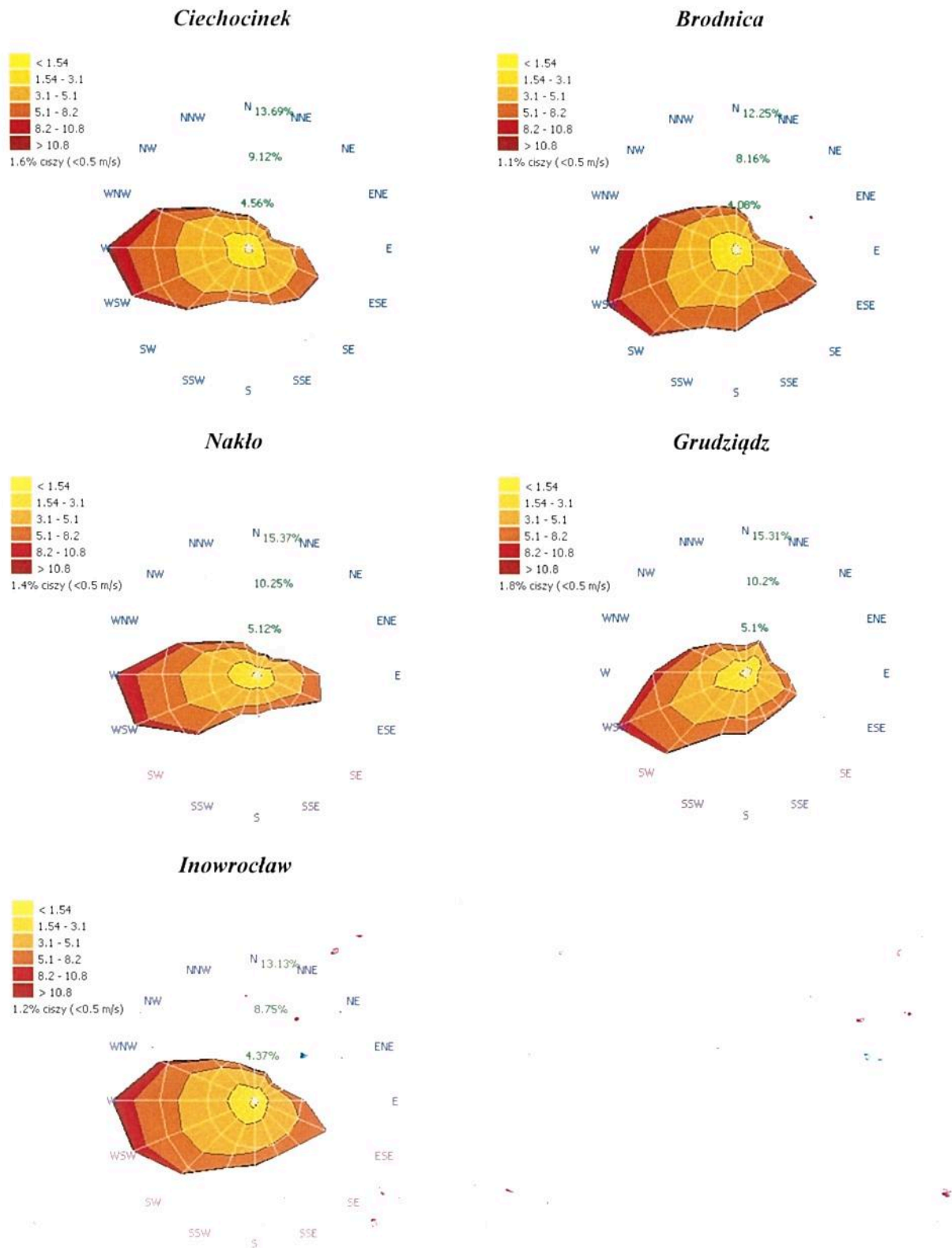
Rysunek 7. Rozkład kierunków i prędkości wiatru na wybranych stanowiskach, wyznaczony przez model WRF/CALMET w strefie kujawsko-pomorskiej w 2015 r.
