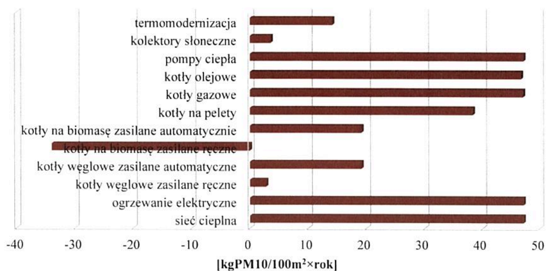
Rysunek 28. Szacunkowy średni efekt ekologiczny działań/inwestycji w postaci wielkości redukcji emisji pyłu zawieszzonego PM10 68
