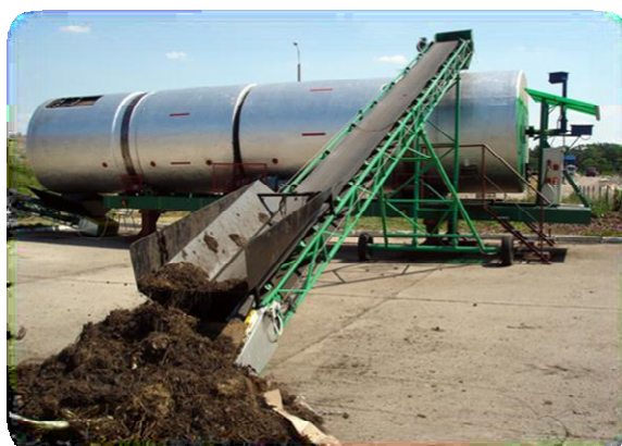
Rysunek 42 Komposter do przetwarzania odpadów zielonych, Machnacz (foto „Saniko” 2013r)
