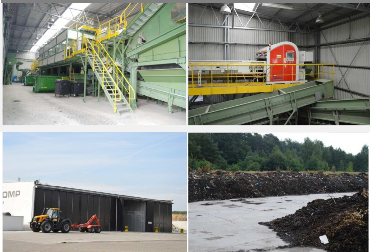
Rysunek 25 Tak jest. Nowa instalacja do biologicznego przetwarzania odpadów z możliwością kompostowania odpadów zielonych, Niedźwiedź (foto: Niedźwiedź, wrzesień 2015r).
