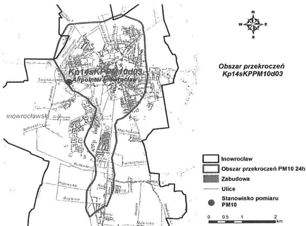
Obszar przekroczeń poziomu dopuszczalnego pyłu zawieszonego PM10 24h Kp14sKPPM10d03 w strefie kujawsko-pomorskiej w 2014 r.
