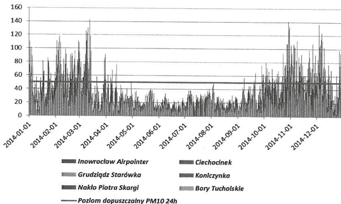
Roczny przebieg średnich dobowych wartości pyłu zawieszonego PM10 na stanowiskach pomiarowych w strefie kujawsko-pomorskiej w 2014 r.
