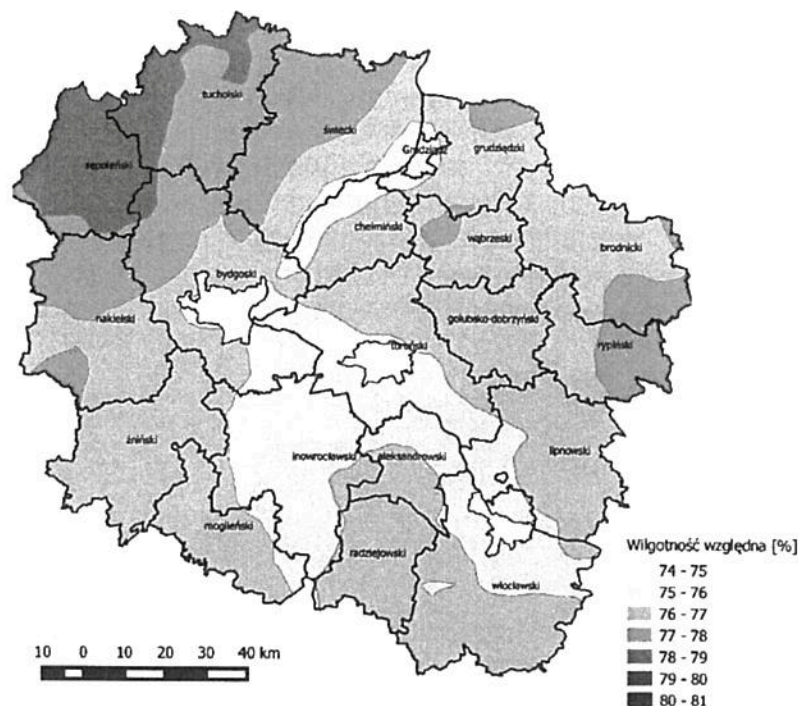
Rozkład średniej rocznej wilgotności względnej powietrza wyznaczonej przez model WRF/CALMET w strefie kujawsko-pomorskiej w 2014 r.
