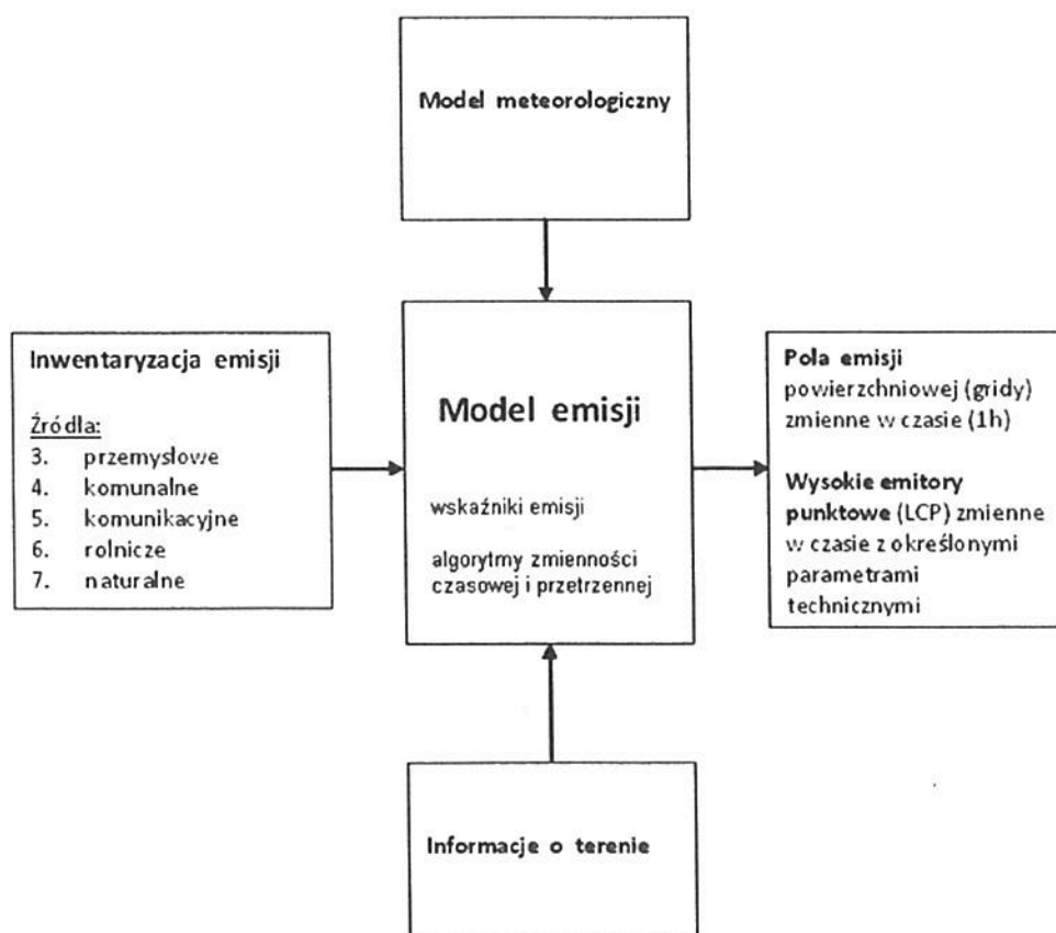
Schemat modelu emisji zanieczyszczeń wykorzystanego w procesie modelowania
