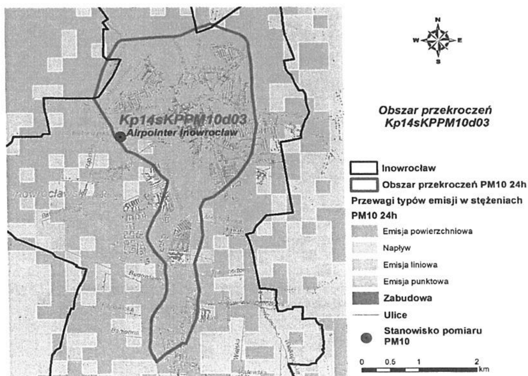
Przewagi typów emisji w stężeniach pyłu zawieszonego PM10 24h w obszarze przekroczeń Kp14sKPPM10d03 w strefie kujawsko-pomorskiej w 2014 r.
