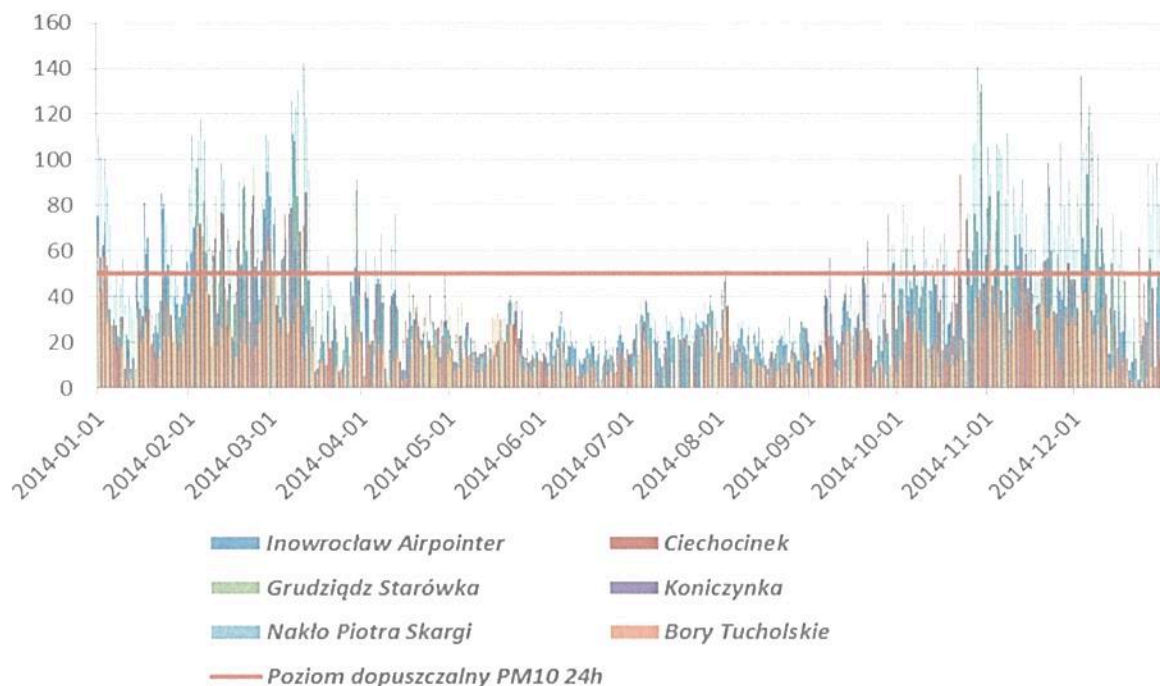
Roczny przebieg średnich dobowych wartości pyłu zawieszonego PM10 na stanowiskach pomiarowych w strefie kujawsko-pomorskiej w 2014 r.
