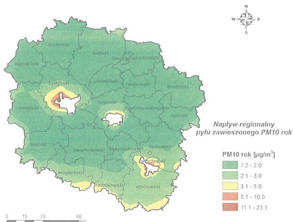
Stężenia pyłu zawieszonego PM10 o okresie uśredniania wyników rok w strefie kujawsko-pomorskiej tworzące tło regionalne w 2014 r.
