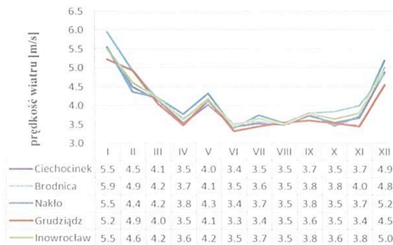
Średnia miesięczna prędkość wiatru wyznaczona przez model WRF/CALMET w strefie kujawsko-pomorskiej w 2014 r.
