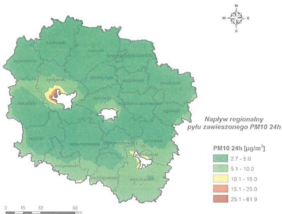
Stężenia pyłu zawieszonego PM10 o okresie uśredniania wyników 24 h w strefie kujawsko-pomorskiej tworzące tło regionalne w 2014 r.
