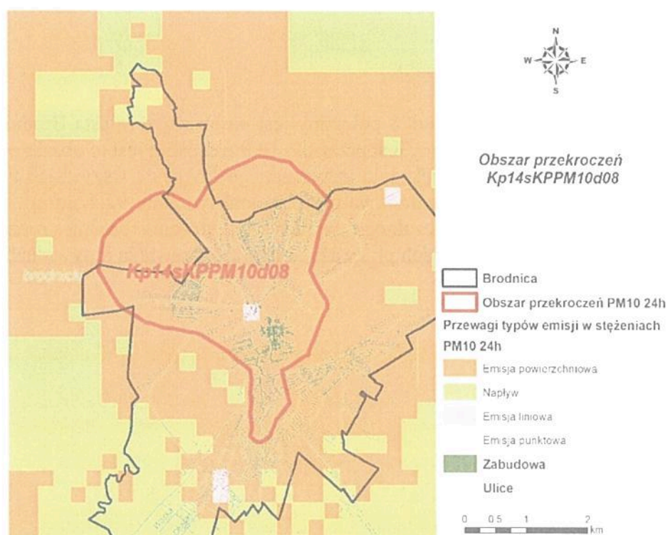
Przewagi typów emisji w stężeniach pyłu zawieszonego PM10 24h w obszarze przekroczeń Kp14sKPPM10d08 w strefie kujawsko-pomorskiej w 2014 r.
