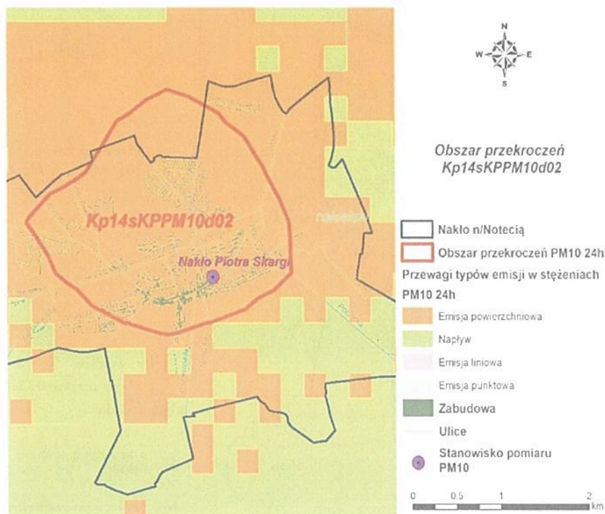
Przewagi typów emisji w stężeniach pyłu zawieszzonego PM10 24h w obszarze przekroczeń Kp14sKPPM10d02 w strefie kujawsko-pomorskiej w 2014 r.
