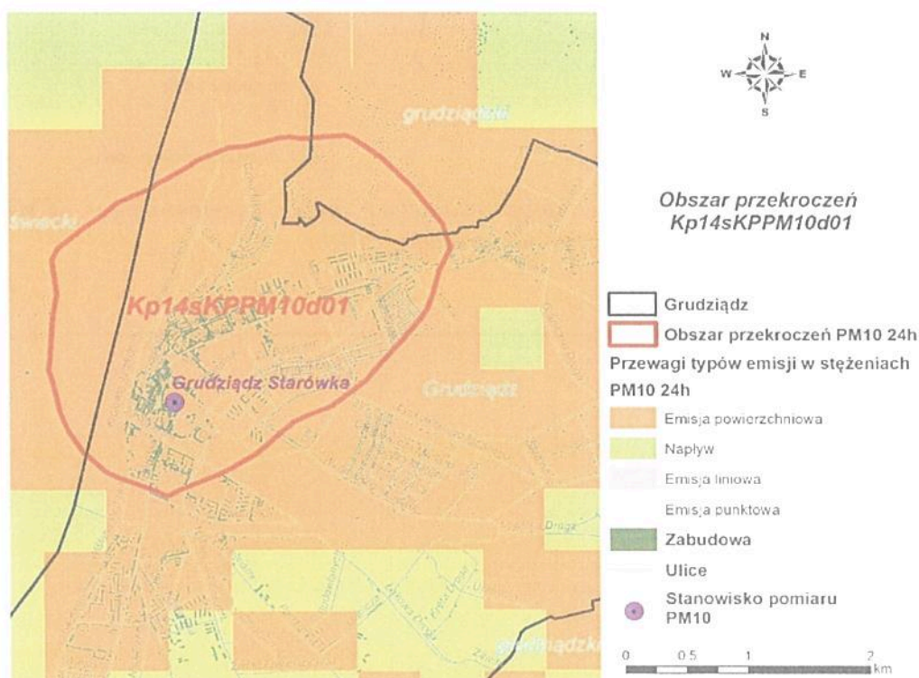
Przewagi typów emisji w stężeniach pyłu zawieszonoego PM10 24h w obszarze przekroczeń Kp14sKPPM10d01 w strefie kujawsko-pomorskiej w 2014 r.
