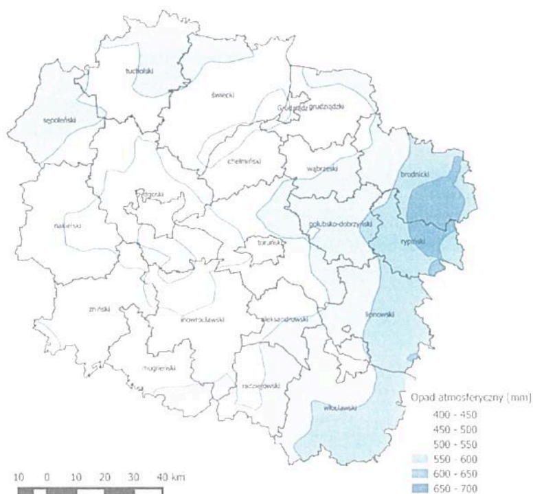
Rozkład rocznej sumy opadów atmosferycznych wyznaczonej przez model WRF/CALMET w strefie kujawsko-pomorskiej w 2014 r.
