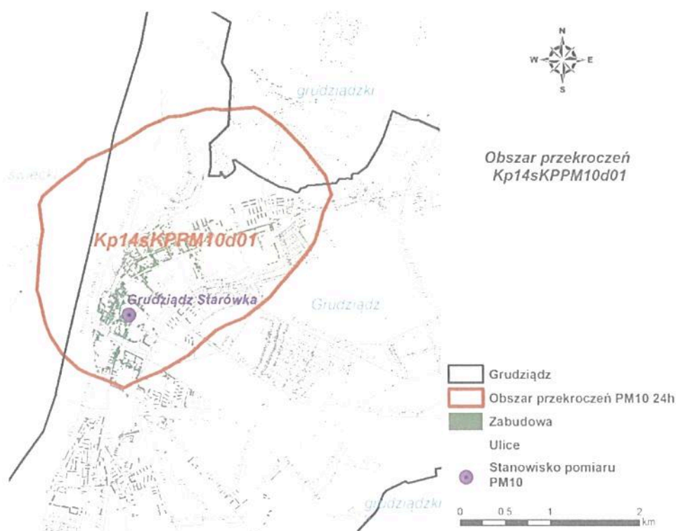
Obszar przekroczeń poziomu dopuszczalnego pyłu zawieszonoego PM10 24h Kp14sKPPM10d01 w strefie kujawsko-pomorskiej w 2014 r.
