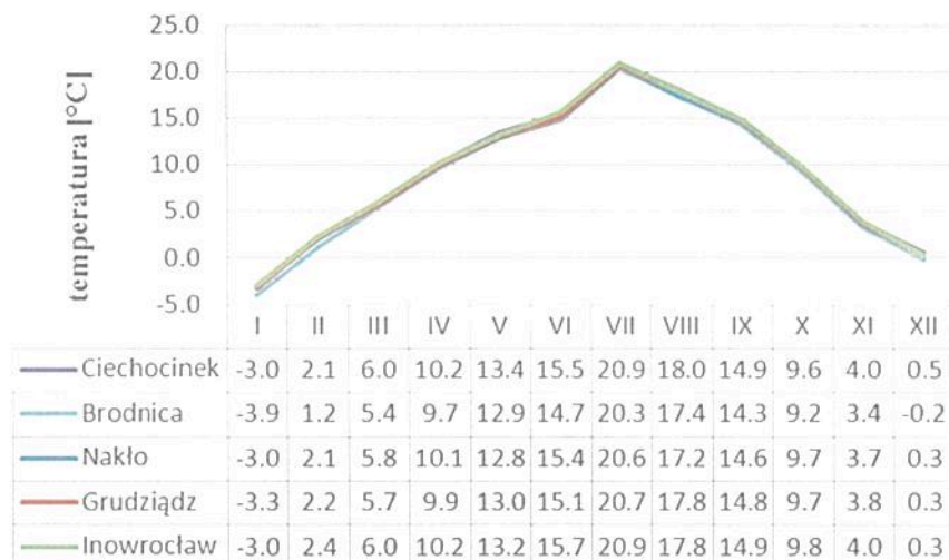
Przebieg średnich miesięcznych wartości temperatury powietrza wyznaczonych przez model WRF/CALMET w strefie kujawsko-pomorskiej w 2014 r.
