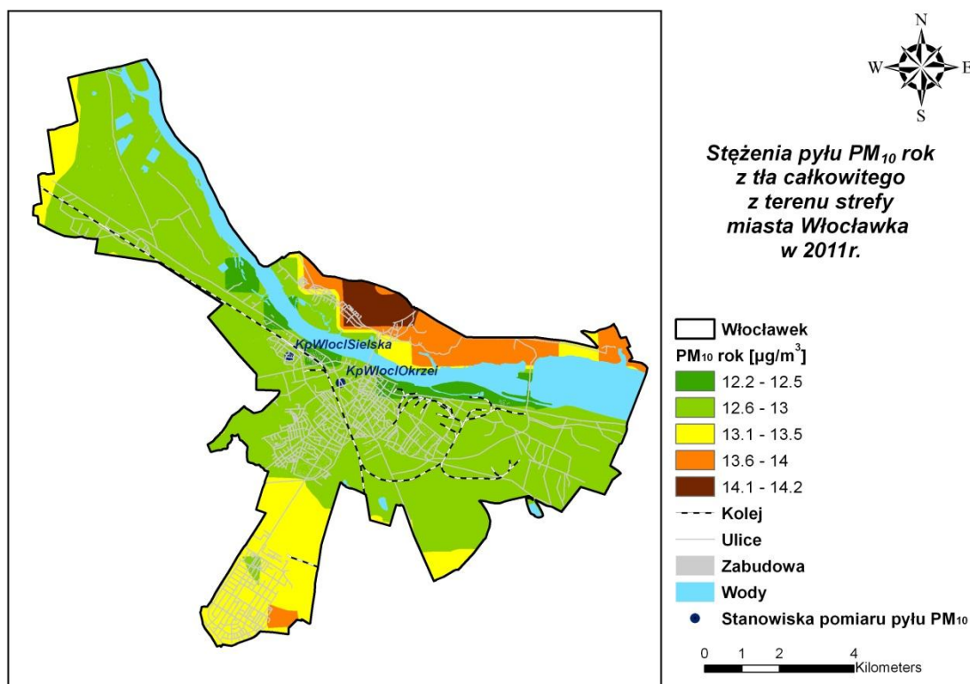
Rysunek 42 Stężenia pyłu PM 10 o okresie uśredniania wyników rok w mieście Włocławek pochodzące z tła całkowitego w 2011 r.
