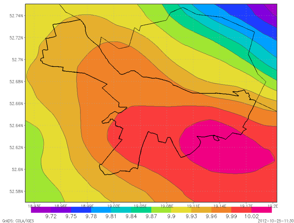
Rysunek 29 Rozkład średniej rocznej wartości temperatury powietrza [°C] w strefie miasto Włocławek w 2011 r.
