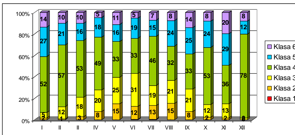
Rysunek 36 Udział klas równowagi atmosfery Pasquilla w strefie miasto Włocławek w 2011 roku
