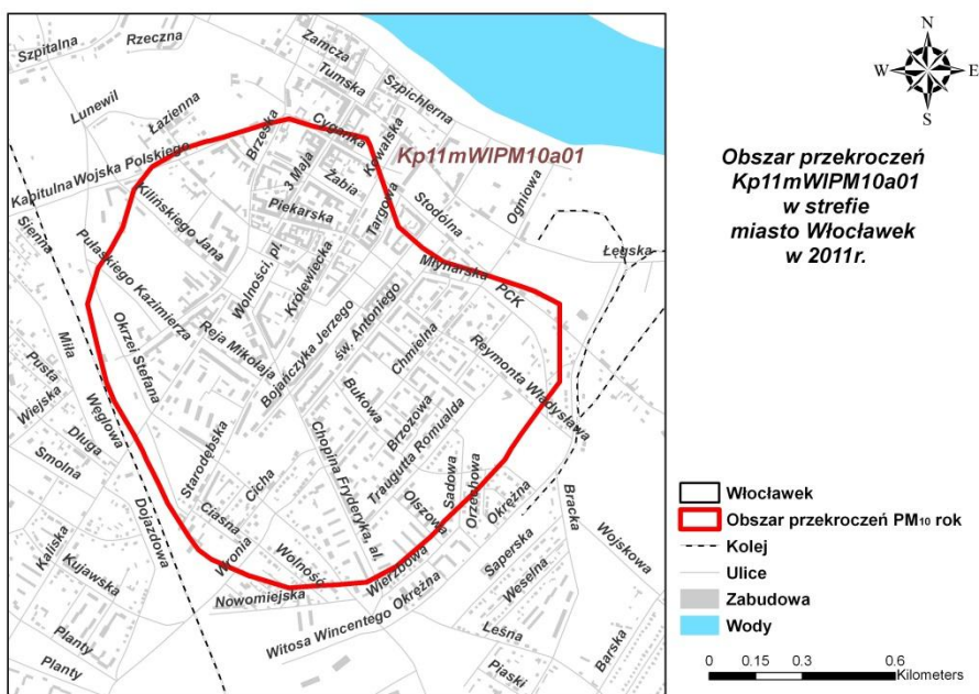
Rysunek 53 Obszar przekroczeń poziomu dopuszczalnego PM 10 rok Kp11mWIPM10a01 w mieście Włocławek w 2011 r.
