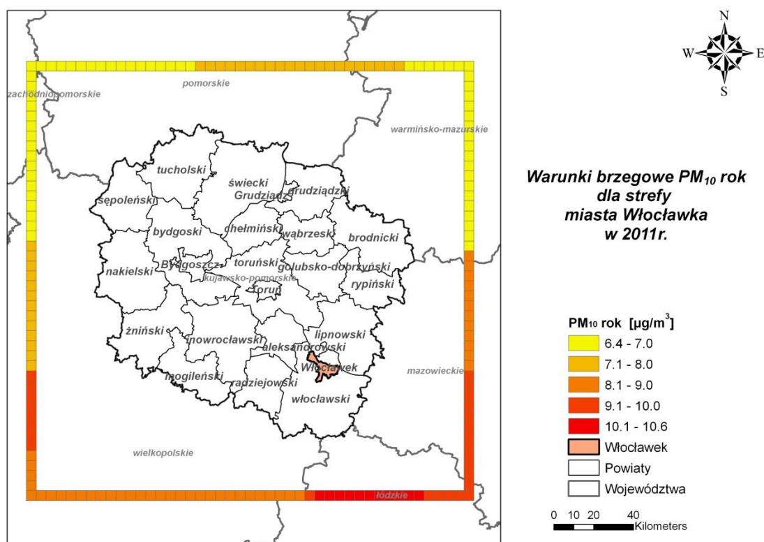
Rysunek 11 Warunki brzegowe pyłu zawieszonego PM 10 dla strefy miasto Włocławek w 2011 r.
