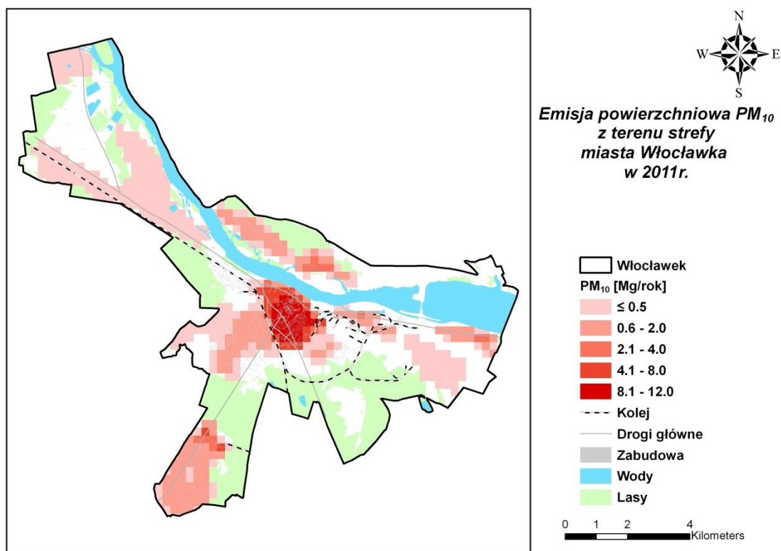
Rysunek 17 Emisja powierzchniowa pyłu PM 10 z terenu miasta Włocławek w 2011 r.
