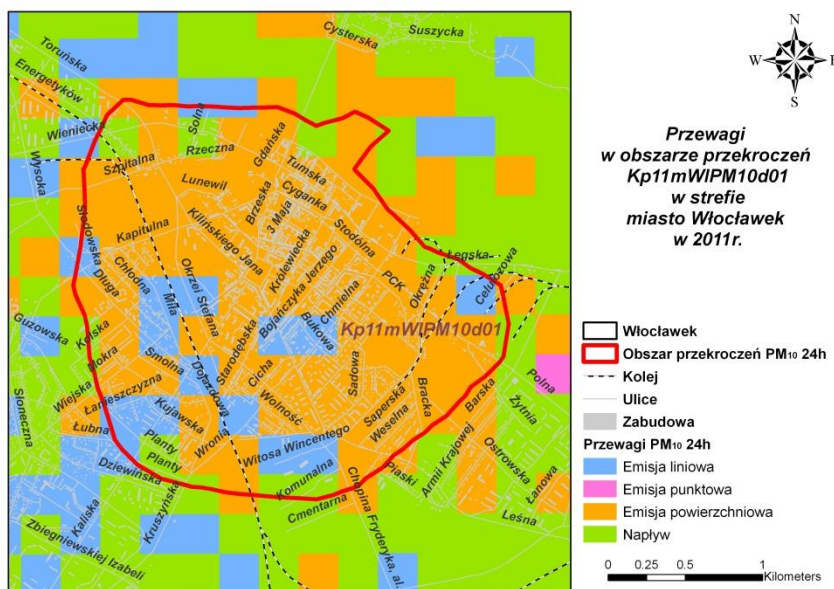
Rysunek 52 Przewagi typów emisji w stężeniach PM 10 24h w obszarze przekroczeń Kp11mWIPM10d01 w mieście Włocławek w 2011 r.
