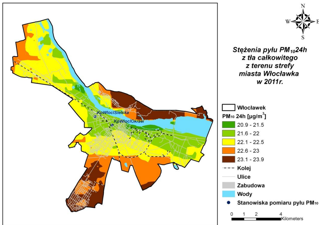
Rysunek 41 Stężenia pyłu PM 10 o okresie uśredniania wyników 24h w mieście Włocławek pochodzące z tła całkowitego w 2011 r.
