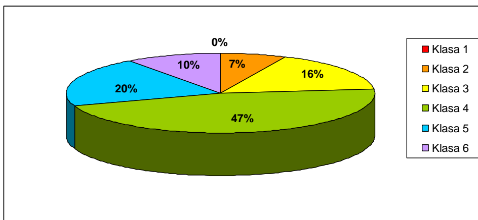
Rysunek 35 Częstość występowania klas równowagi atmosfery Pasquilla w strefie miasto Włocławek w 2011 r.
