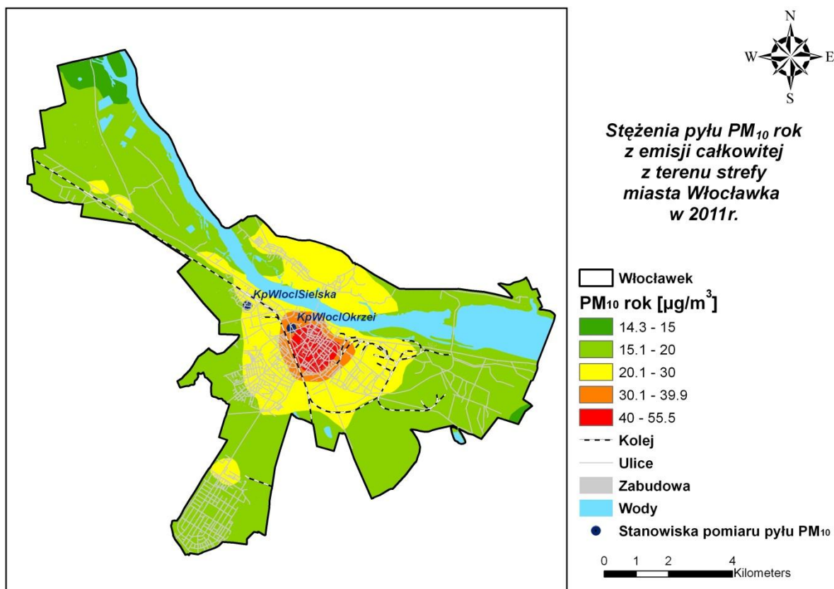
Rysunek 50 Stężenia pyłu PM 10 o okresie uśredniania wyników rok w mieście Włocławek pochodzące z łącznej emisji wszystkich typów w 2011 r.
