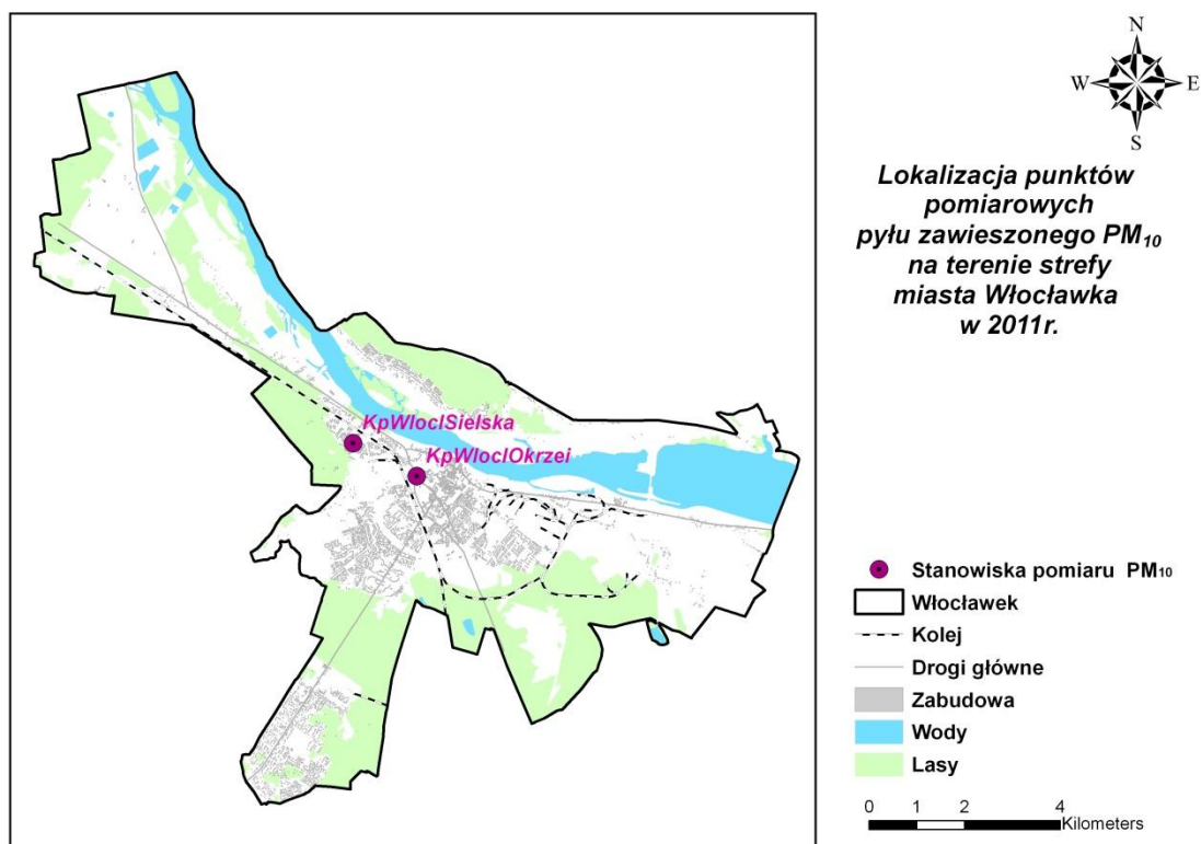
Rysunek 3 Lokalizacja stanowisk pomiarowych PM 10 w strefie miasto Włocławek
