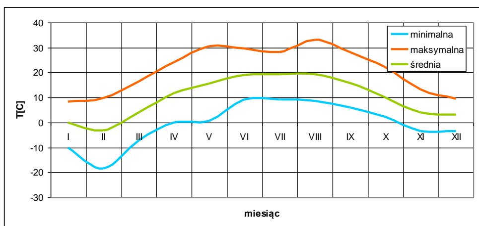
Rysunek 28 Przebieg średnich miesięcznych wartości temperatury powietrza w strefie miasto Włocławek w 2011 r.
