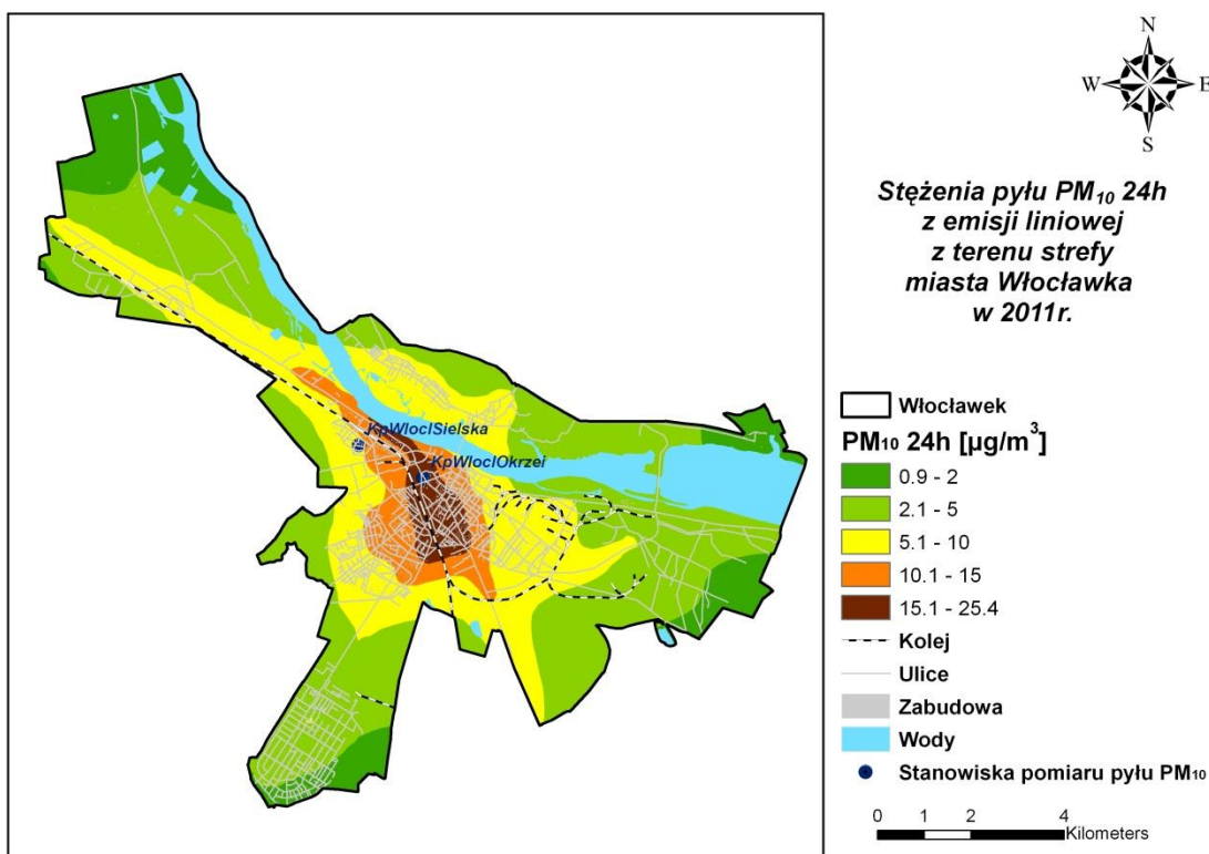
Rysunek 47 Stężenia pyłu PM 10 o okresie uśredniania wyników 24h w mieście Włocławek pochodzące z emisji komunikacyjnej w 2011 r.
