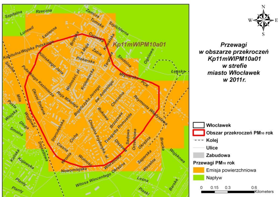
Rysunek 54 Przewagi typów emisji w stężeniach PM 10 rok w obszarze przekroczeń Kp11mWIPM10a01 w mieście Włocławek w 2011 r.
