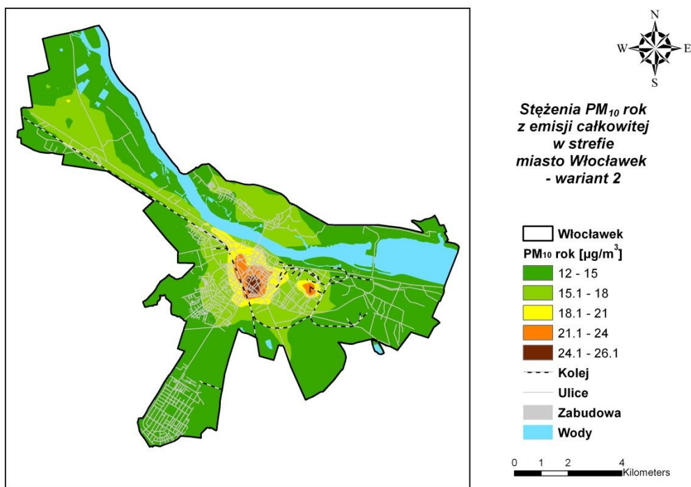
Rysunek 56 Stężenia pyłu PM 10 o okresie uśredniania wyników rok w mieście Włocławek pochodzące z łącznej emisji wszystkich typów po zastosowaniu wariantu naprawczego
