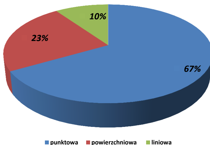
Rysunek 15 Udział procentowy emisji pyłu PM 10 poszczególnych typów z miasta Włocławek w 2011 r.
