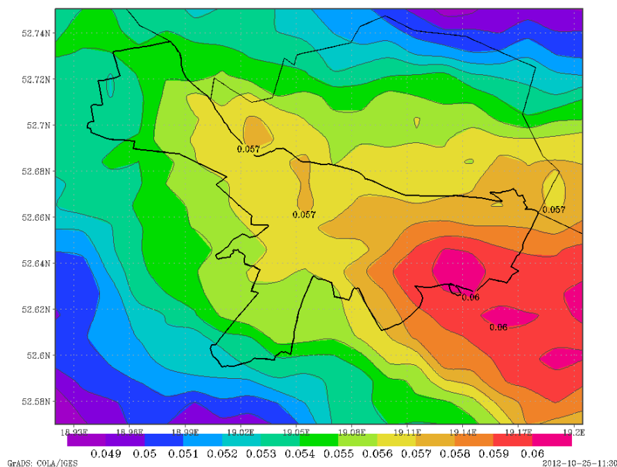
Rysunek 27 Rozkład częstości występowania ciszy atmosferycznej i wiatrów o małej prędkości w strefie miasto Włocławek w 2011 r.
