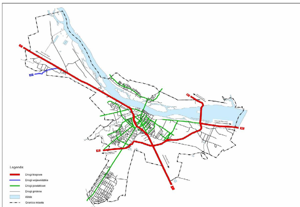
Rysunek 13 Układ komunikacyjny Włocławka
