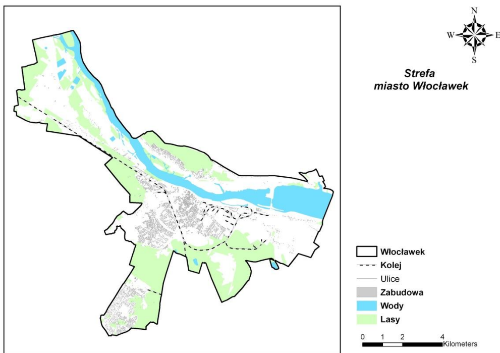
Rysunek 58 Strefa miasto Włocławek
