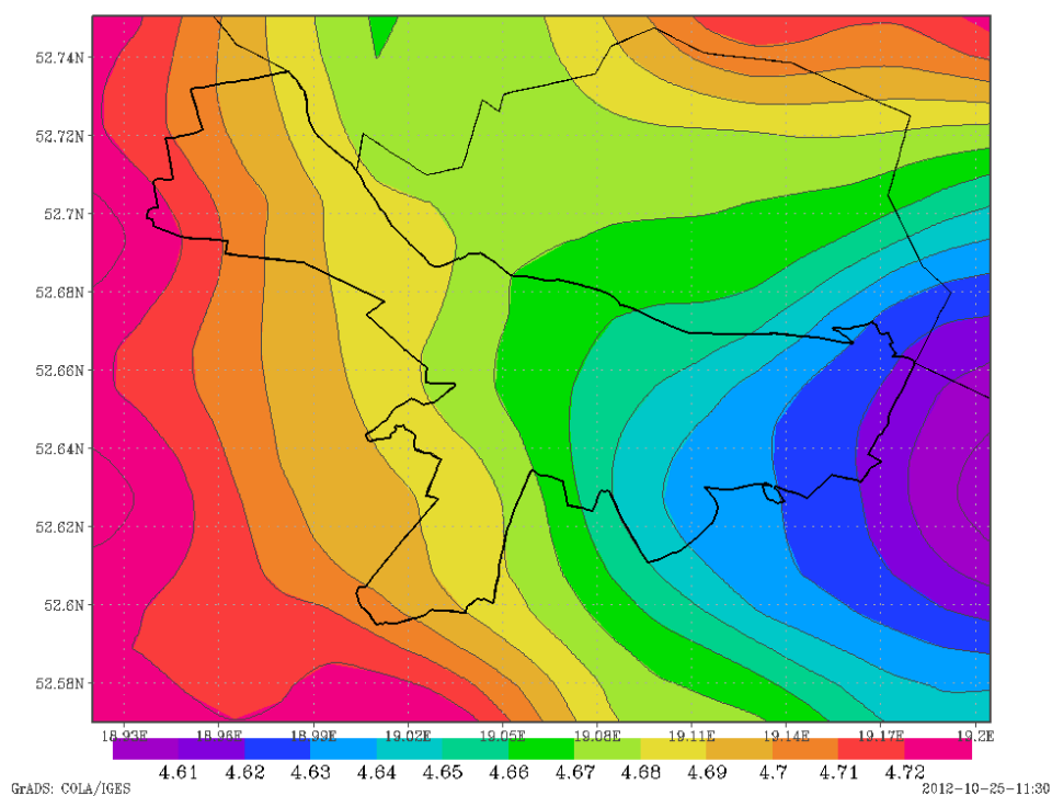
Rysunek 23 Rozkład średniej rocznej wartości prędkości wiatru [m/s] w strefie miasto Włocławek w 2011r.
