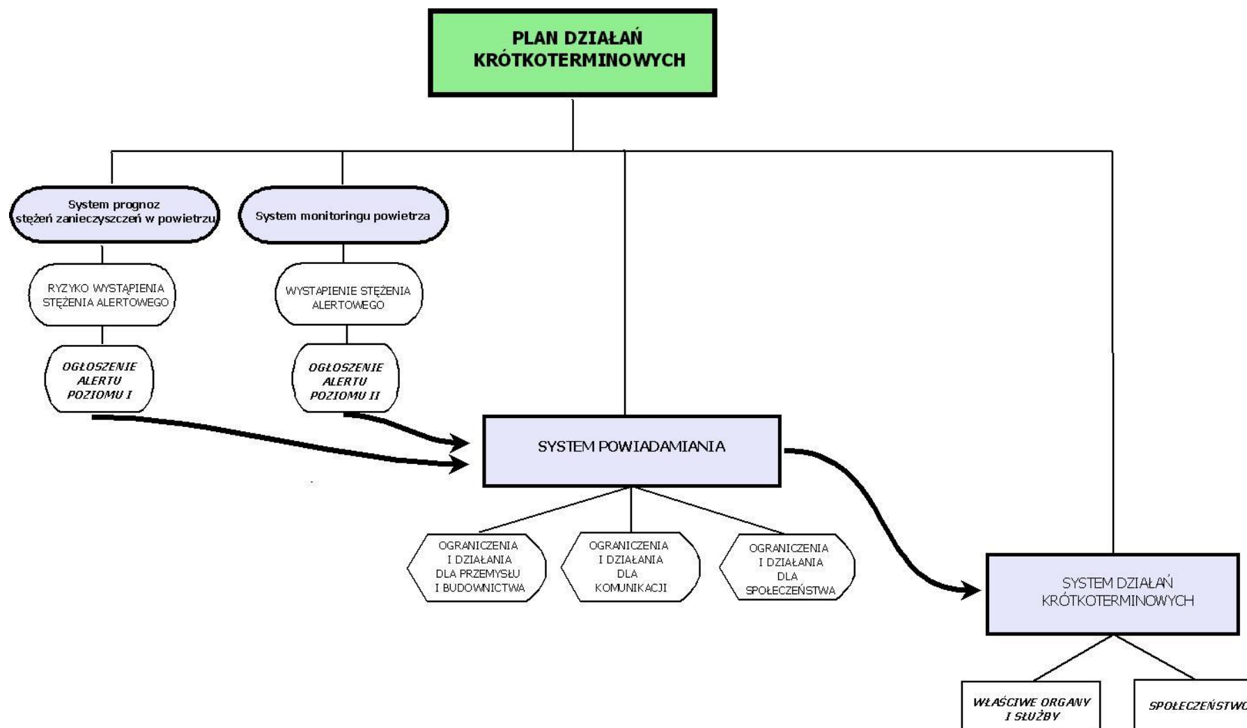
Rysunek 57 Plan działań krótkoterminowych
