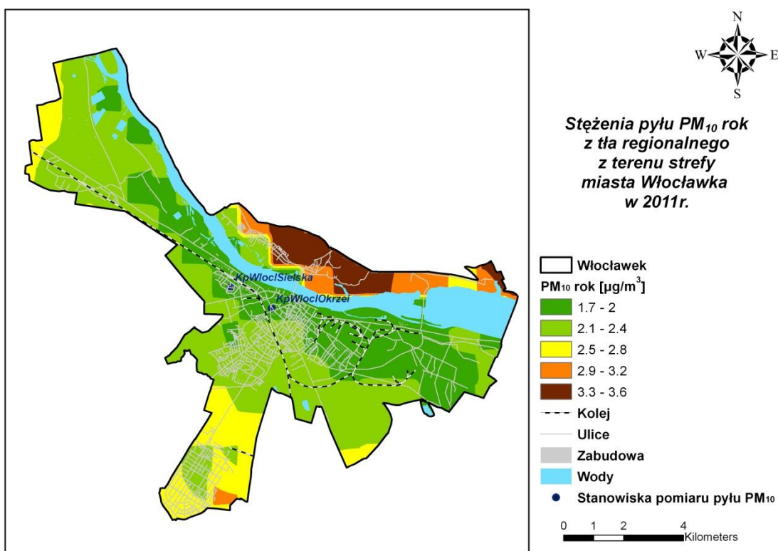
Rysunek 40 Stężenia pyłu PM 10 o okresie uśredniania wyników rok w mieście Włocławek pochodzące z tła regionalnego w 2011 r.
