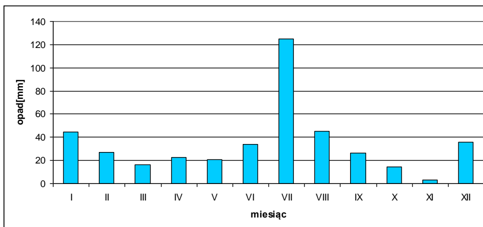
Rysunek 31 Miesięczne sumy opadu atmosferycznego w strefie miasto Włocławek w 2011 r.
