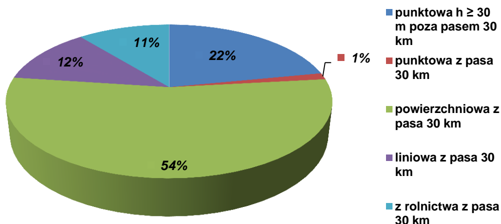
Rysunek 14 Udział procentowy emisji napływowej pyłu PM 10 dla miasta Włocławek w 2011 r.
