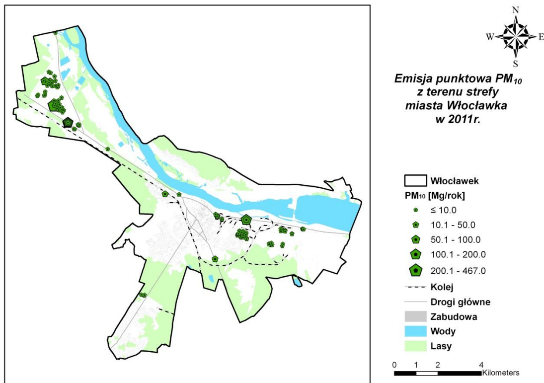
Rysunek 16 Emisja punktowa pyłu PM 10 z terenu miasta Włocławek w 2011 r.
