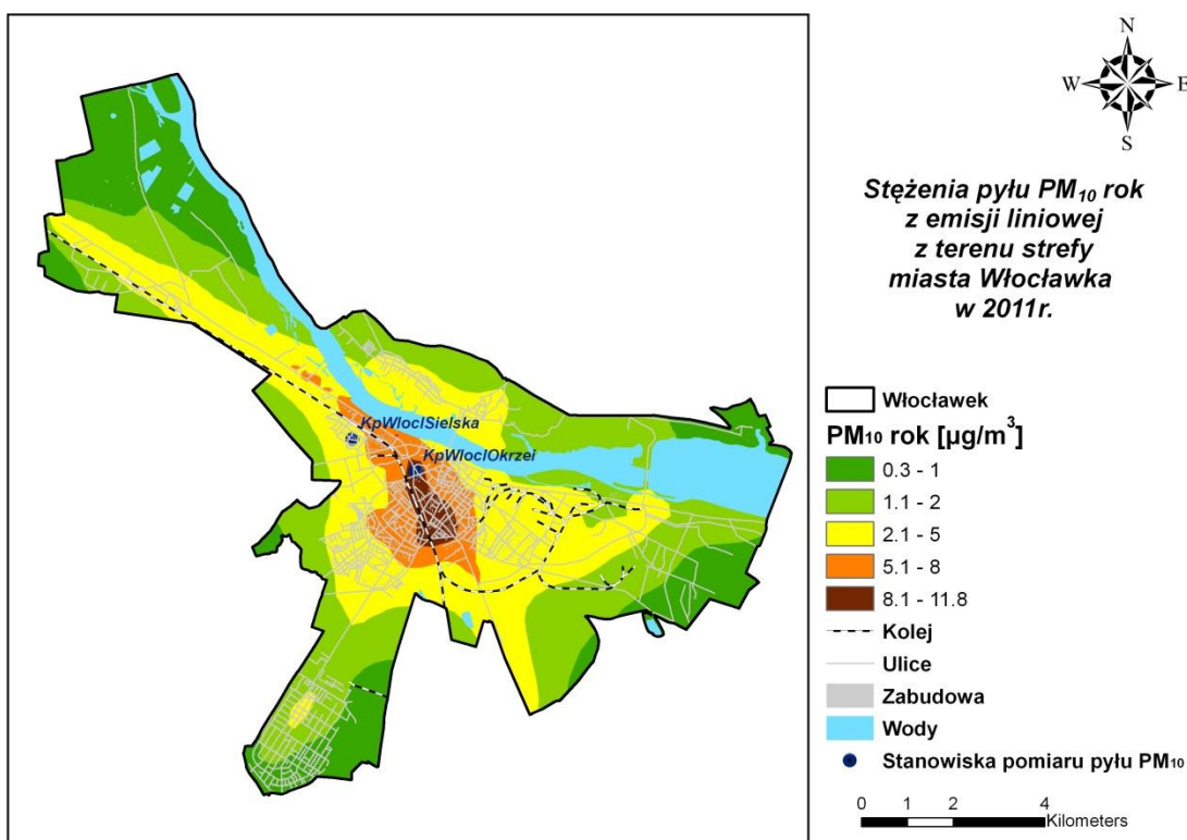
Rysunek 48 Stężenia pyłu PM 10 o okresie uśredniania wyników rok w mieście Włocławek pochodzące z emisji komunikacyjnej w 2011 r.
