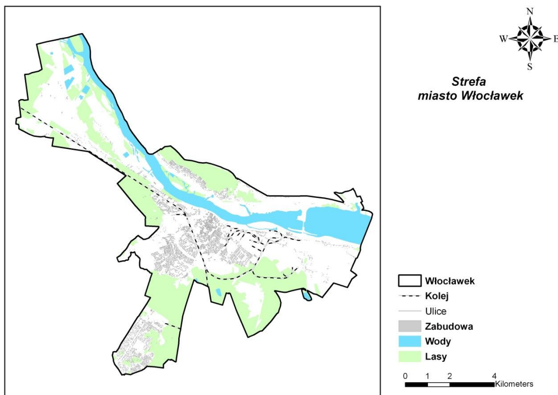
Rysunek 2 Strefa miasto Włocławek
