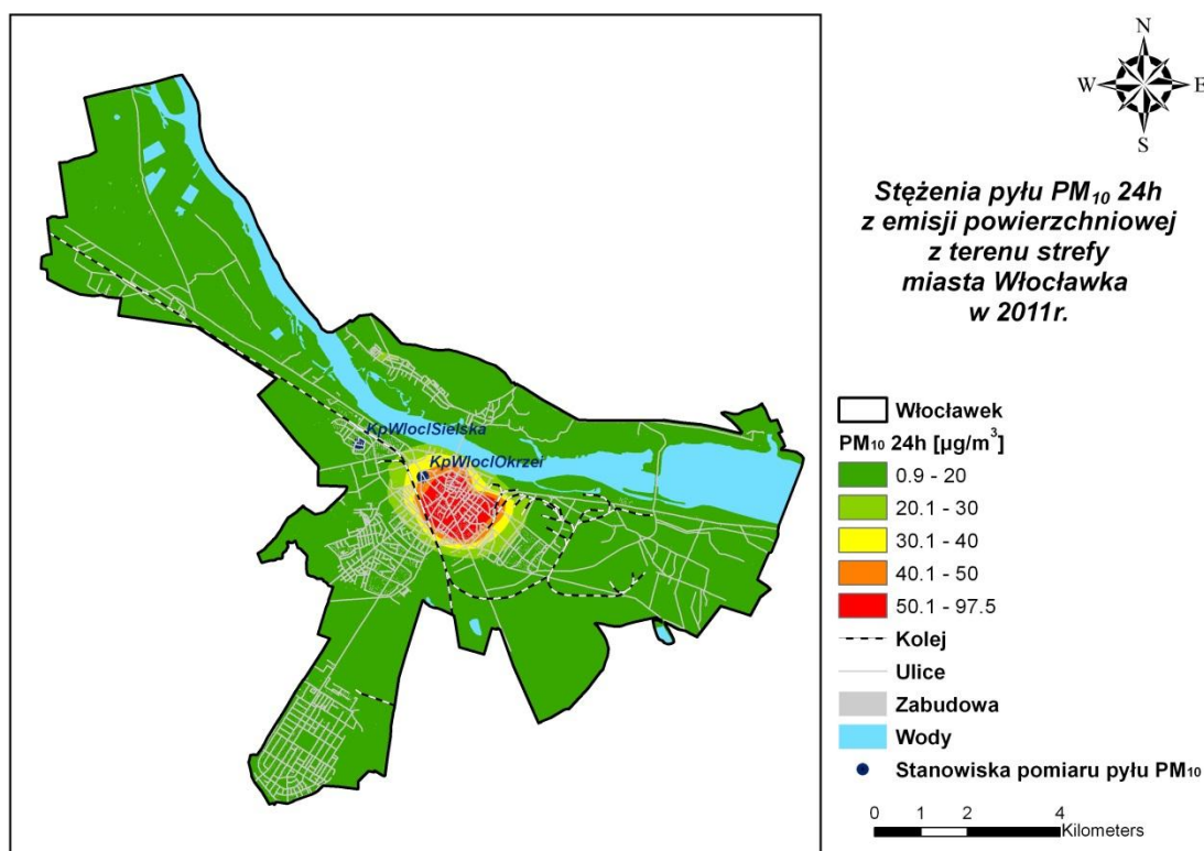
Rysunek 45 Stężenia pyłu PM 10 o okresie uśredniania wyników 24h w mieście Włocławek pochodzące z emisji komunalnej w 2011 r.
