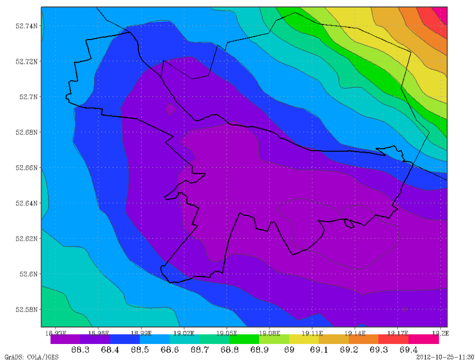
Rysunek 32 Rozkład średniej rocznej wartości wilgotności powietrza atmosferycznego w strefie miasto Włocławek w 2011 r.
