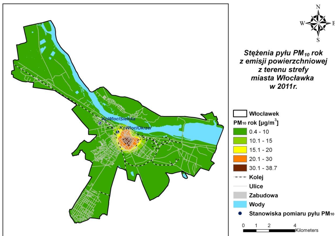
Rysunek 46 Stężenia pyłu PM 10 o okresie uśredniania wyników rok w mieście Włocławek pochodzące z emisji komunalnej w 2011 r.
