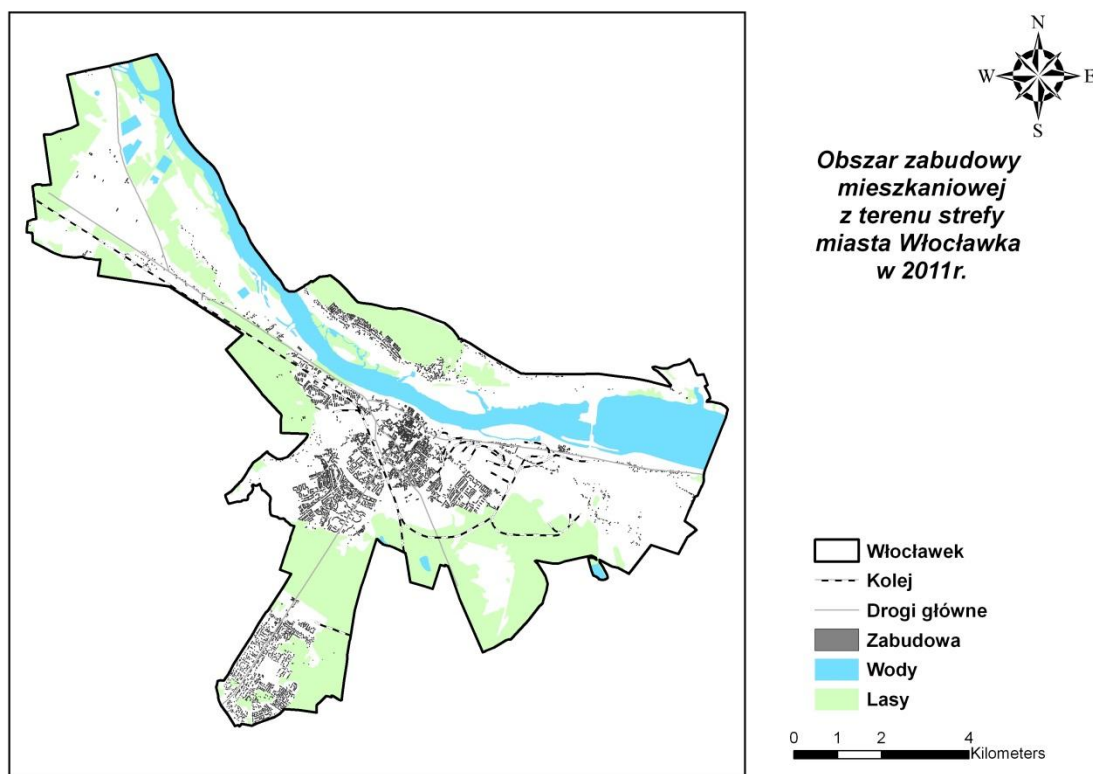
Rysunek 12 Obszar zabudowy mieszkaniowej we Włocławku
