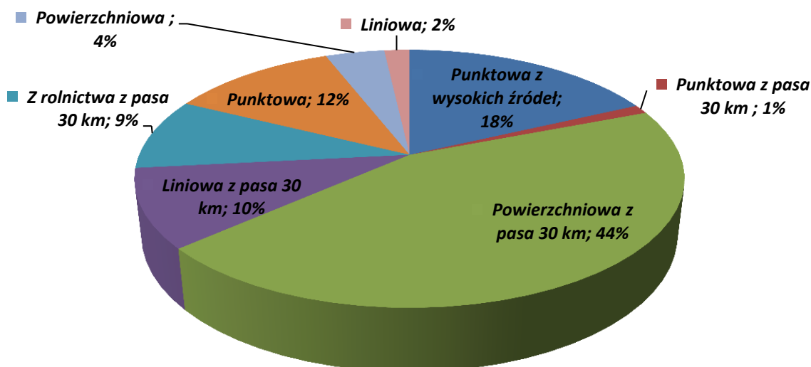
Rysunek 22 Procentowy udział typów źródeł w bilansie emisji dla strefy miasto Włocławek w 2011 r.
