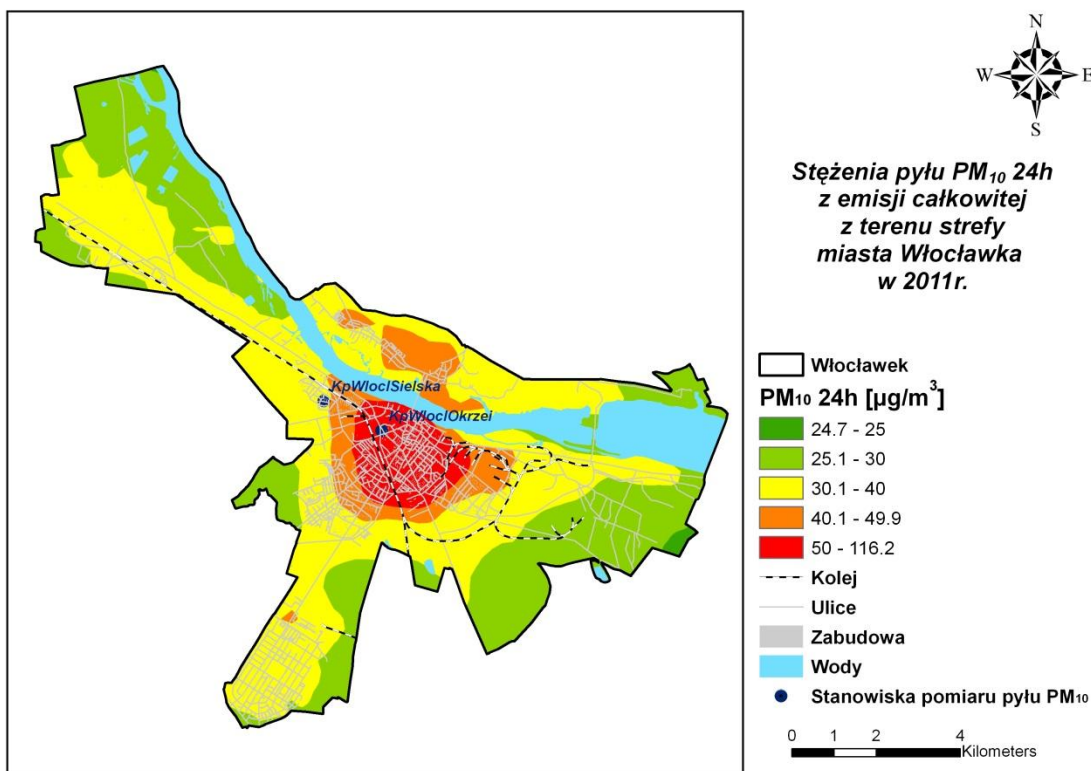
Rysunek 49 Stężenia pyłu PM 10 o okresie uśredniania wyników 24h w mieście Włocławek pochodzące z łącznej emisji wszystkich typów w 2011 r.
