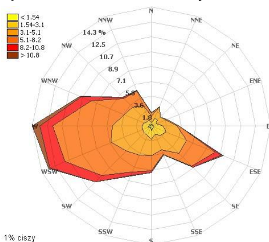
Rysunek 25 Róża wiatrów dla strefy miasto Włocławek – sezon zimowy w 2011 r.
