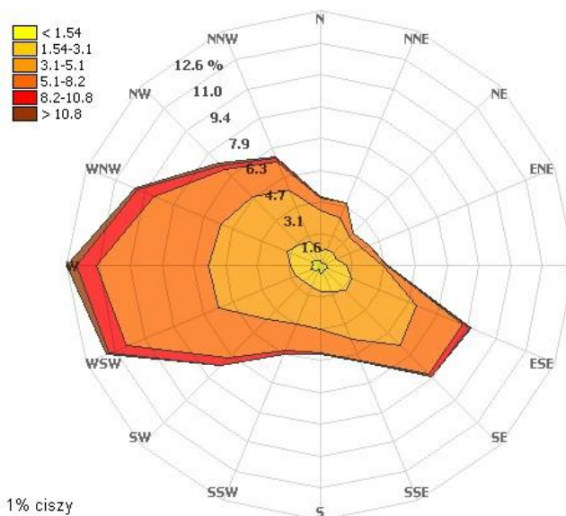
Rysunek 24 Róża wiatrów dla strefy miasto Włocławek w 2011 r.
