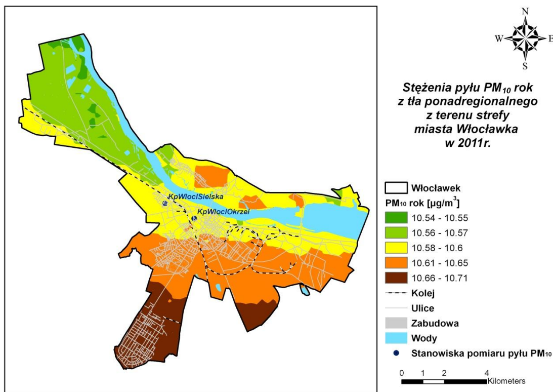
Rysunek 38 Stężenia pyłu PM 10 o okresie uśredniania wyników rok w mieście Włocławek pochodzące z tła ponadregionalnego w 2011 r.
