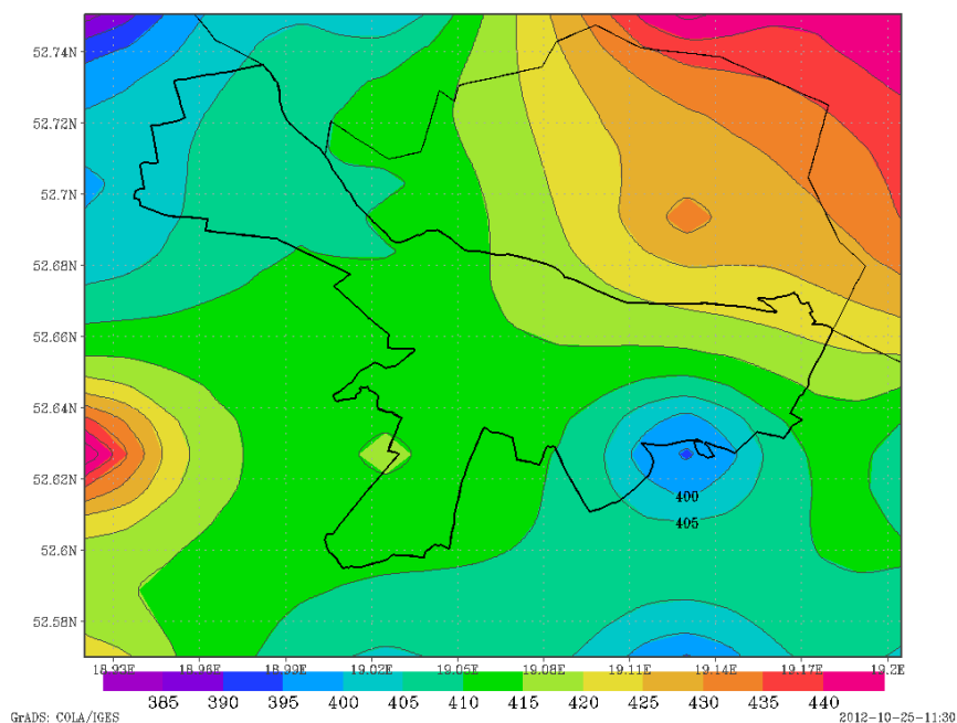
Rysunek 30 Rozkład rocznej sumy opadu atmosferycznego [mm] w strefie miasto Włocławek w 2011 r.
