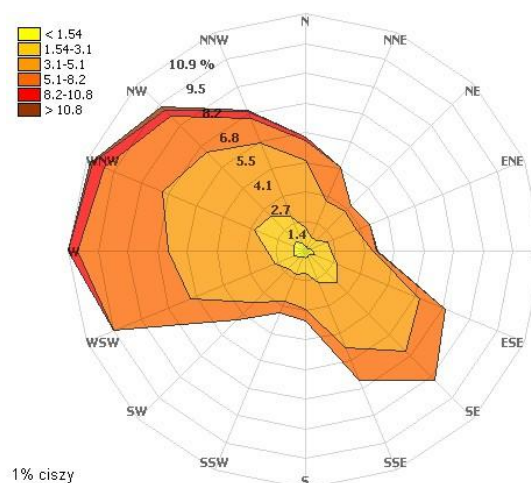
Rysunek 26 Róża wiatrów dla strefy miasto Włocławek – sezon letni w 2011 r.
