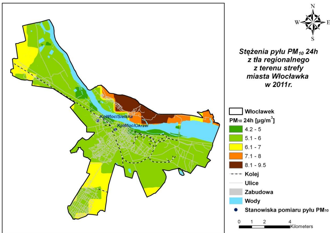
Rysunek 39 Stężenia pyłu PM 10 o okresie uśredniania wyników 24h w mieście Włocławek pochodzące z tła regionalnego w 2011 r.
