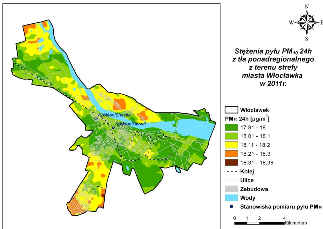
Rysunek 37 Stężenia pyłu PM 10 o okresie uśredniania wyników 24h w mieście Włocławek pochodzące z tła ponadregionalnego w 2011 r.
