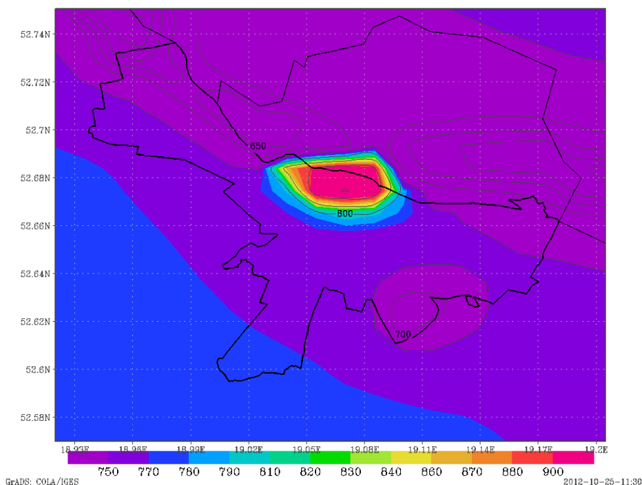
Rysunek 33 Rozkład średniej miesięcznej miąższości warstwy mieszania w strefie miasto Włocławek w roku 2011.
