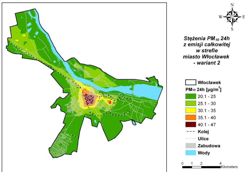
Rysunek 55 Stężenia pyłu PM 10 o okresie uśredniania wyników 24h w mieście Włocławek pochodzące z łącznej emisji wszystkich typów po zastosowaniu wariantu naprawczego
