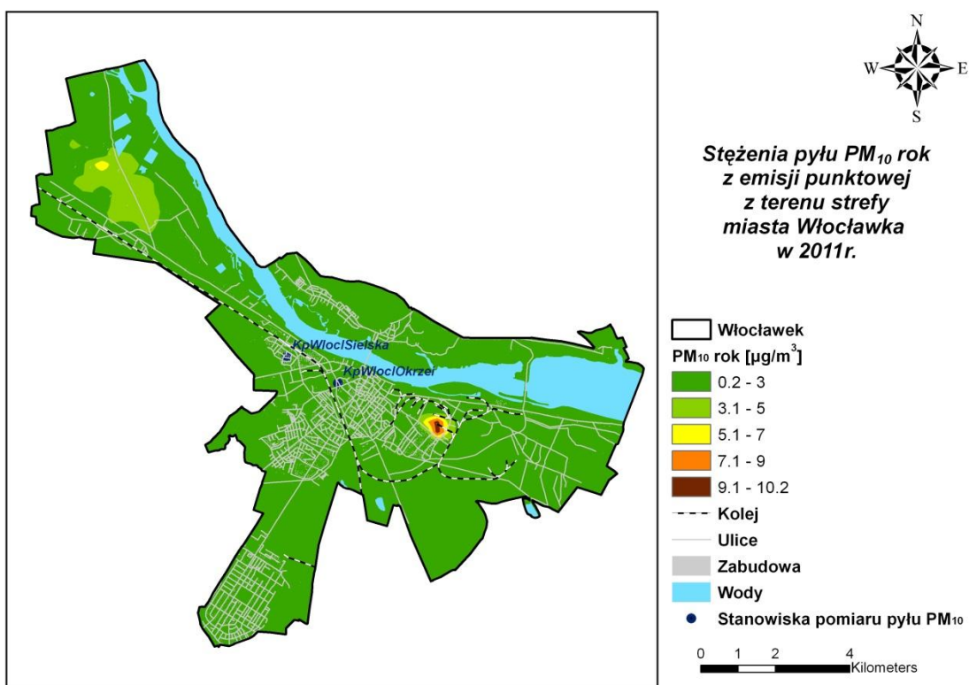
Rysunek 44 Stężenia pyłu PM 10 o okresie uśredniania wyników rok w mieście Włocławek pochodzące z emisji punktowej w 2011 r.
