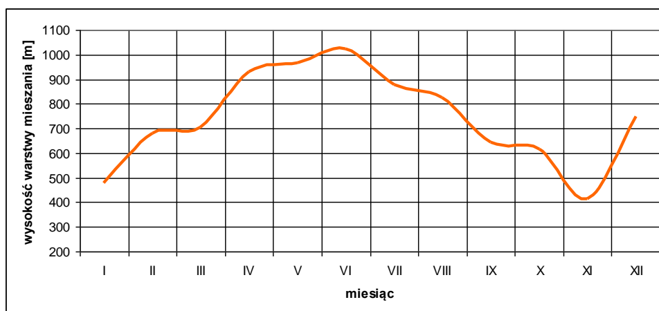
Rysunek 34 Przebieg średnich miesięcznych wartości miąższości warstwy mieszania w strefie miasto Włocławek w 2011 r.
