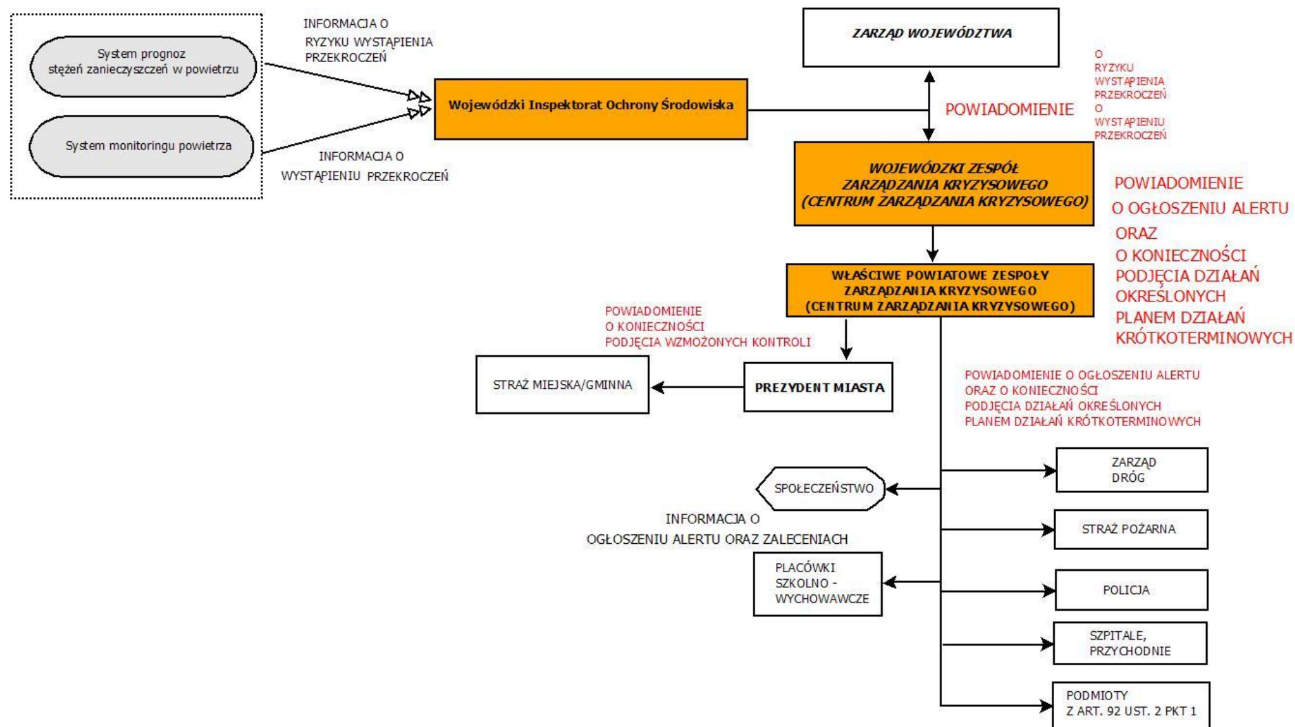
Rysunek 59 Schemat przepływu informacji w Planie Działań Krótkoterminowych
