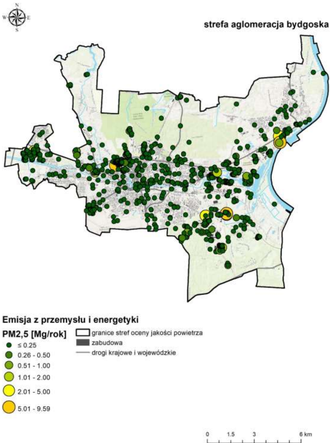
Rysunek 44. Emisja pyłu zawieszonego PM 2,5 z przemysłu i energetyki w 2018 r. 129
