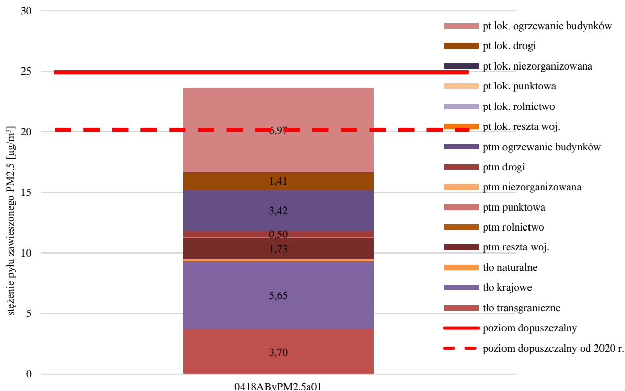
Rysunek 23. Prezentacja poziomów tła regionalnego oraz przyrostu tła lokalnego na terenie obszarów przekroczeń pyłu \text{PM}_{2,5} w strefie aglomeracji bydgoskiej w 2018 roku 83
