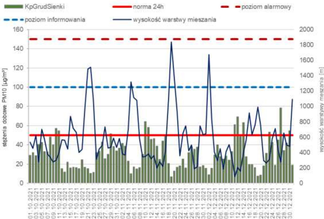
Rysunek 12. Porównanie przebiegu zmienności stężeń 24-godz. PM10 w IV kwartale 2021 r. w Grudziądzu z wysokością warstwy mieszaną 49
