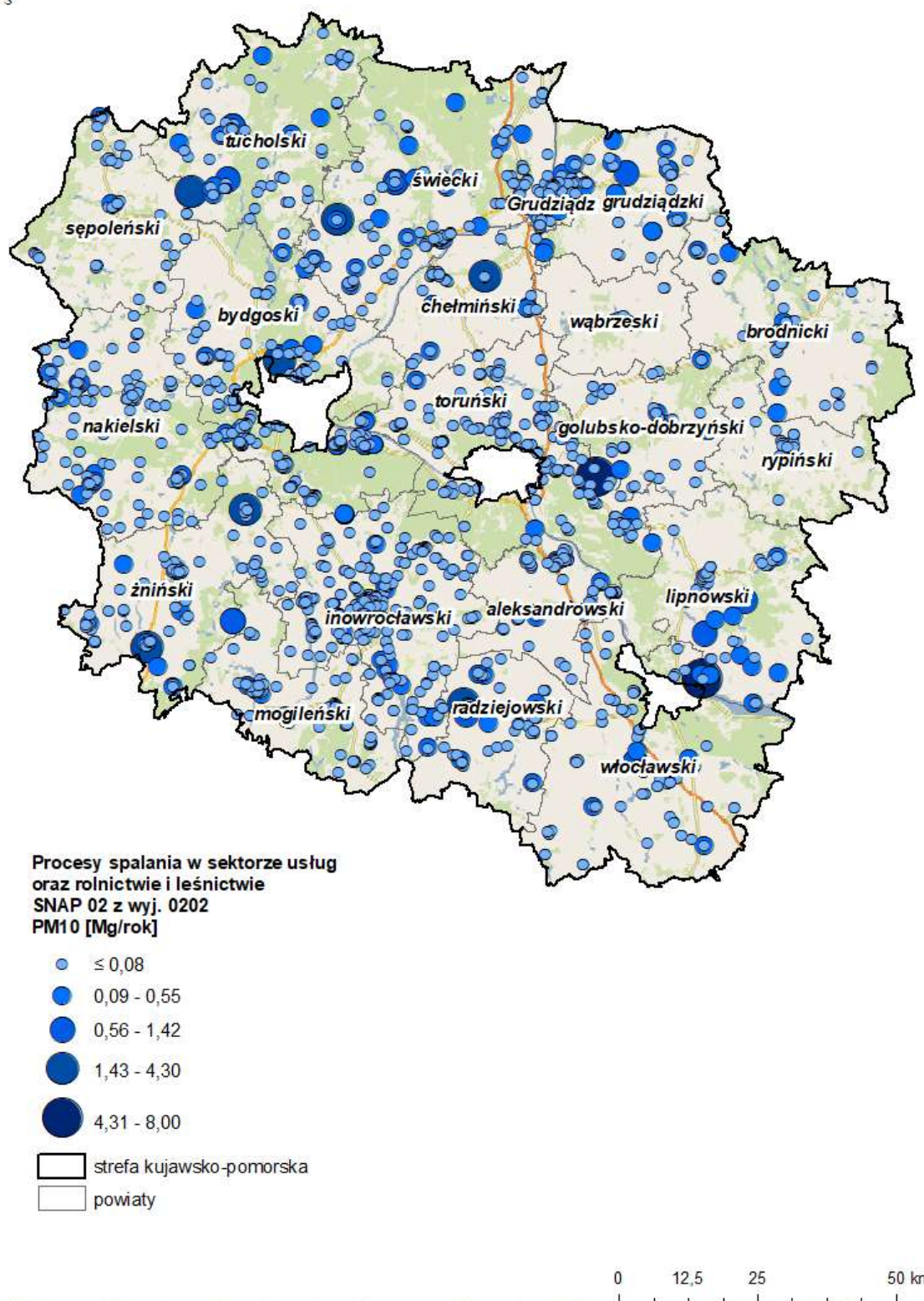
Rysunek 25. Emisja pyłu zawieszonego PM10 z procesów spalania w sektorze usług oraz rolnictwie i leśnictwie (SNAP 02 z wyj. 0202) w 2021 roku 104
