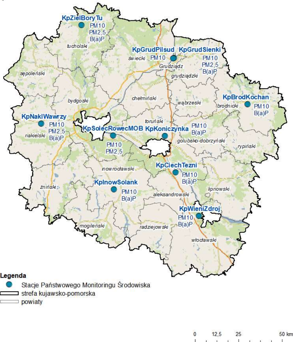
Rysunek 23. Lokalizacja punktów pomiarowych w strefie kujawsko-pomorskiej 102
