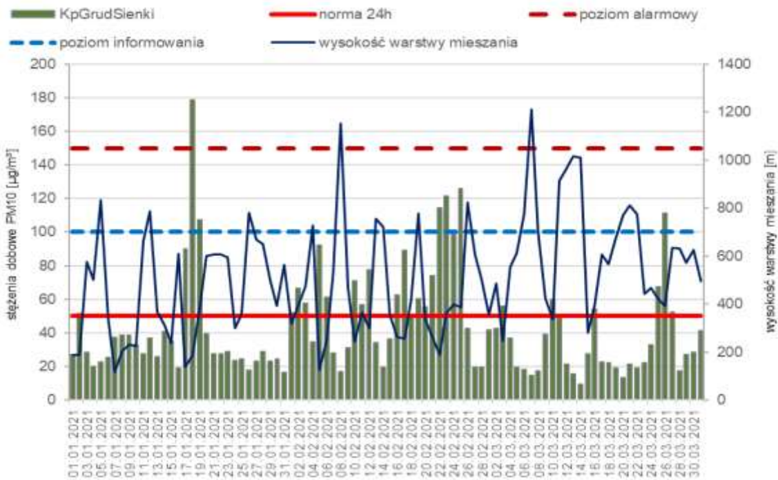
Rysunek 11. Porównanie przebiegu zmienności stężeń 24-godz. PM10 w I kwartale 2021 r. w Grudziądzu z wysokością warstwy mieszaną 48
