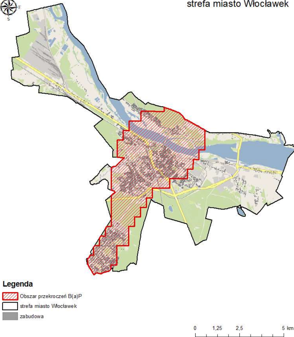
Rysunek 17. Obszar przekroczeń poziomu docelowego dla benzo(a)pirenu, na terenie strefy miasto Włocławek w 2021 roku 64
