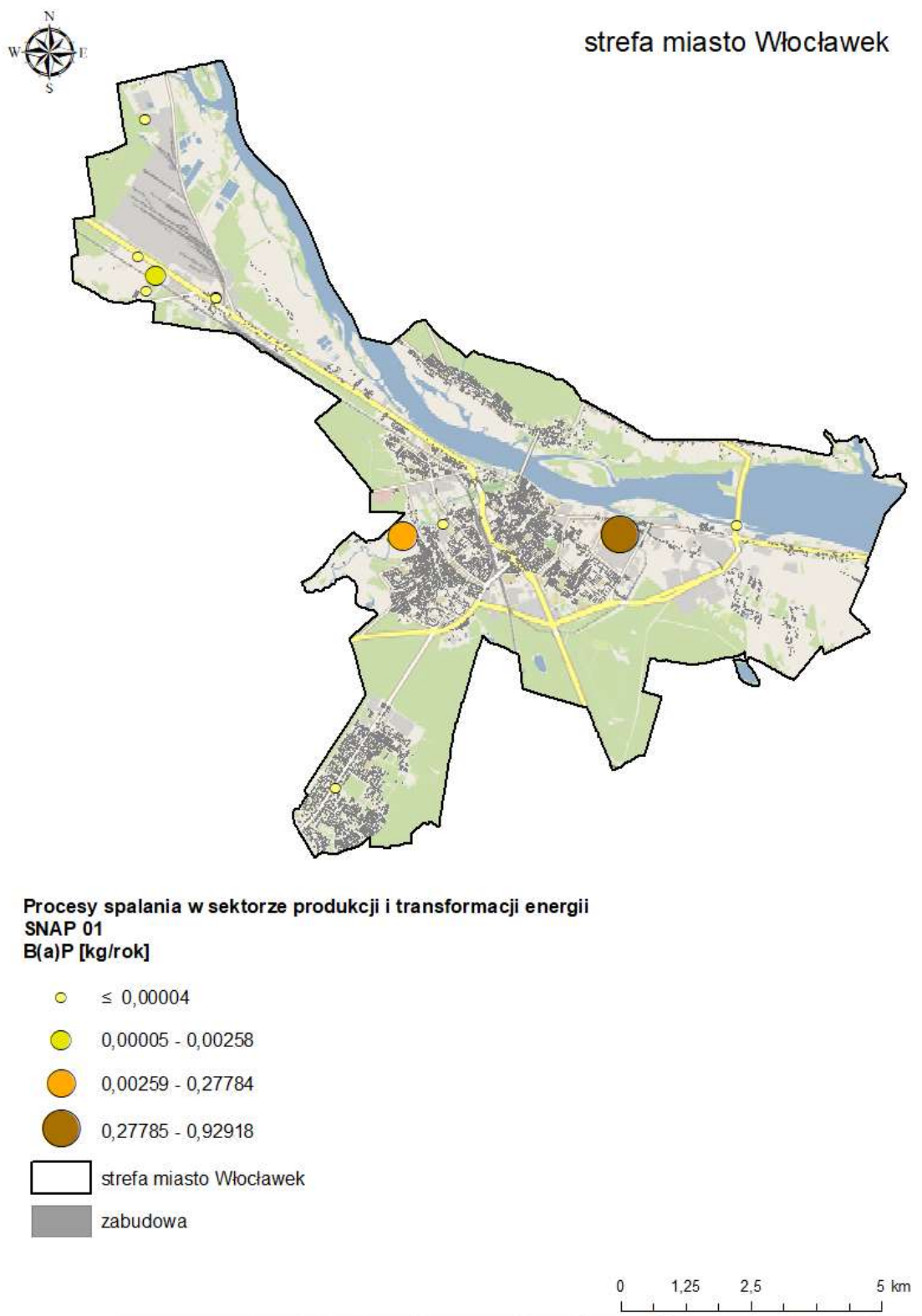
Rysunek 43. Emisja benzo(a)pirenu z procesów spalania w sektorze produkcji i transformacji energii (SNAP 01) 121
