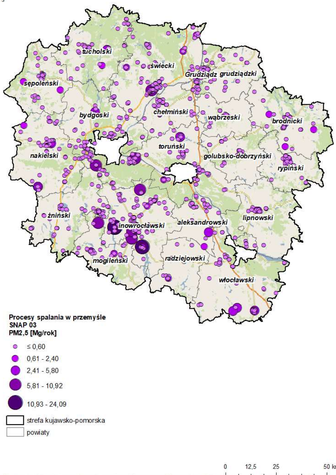
Rysunek 38. Emisja pyłu zawieszonego PM 2,5 z procesów spalania w przemyśle (SNAP 03) w 2021 roku 119
