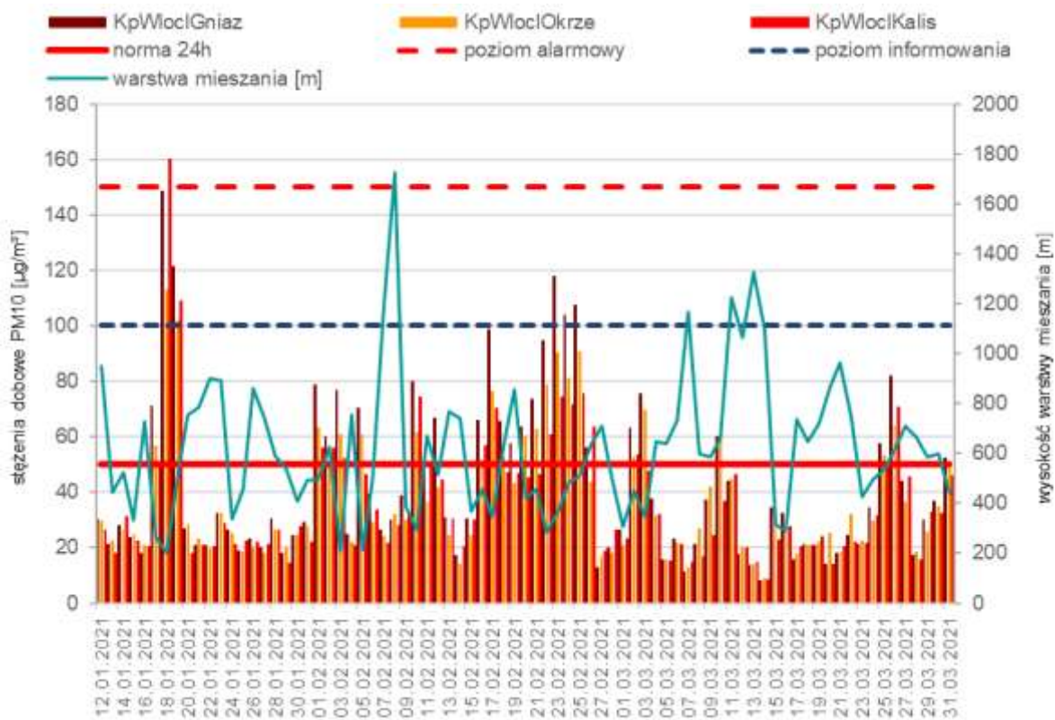
Rysunek 11. Porównanie przebiegu zmienności stężeń 24-godz. PM10 w I kwartale 2021 r. we Włocławku z wysokością warstwy mieszanicy 52
