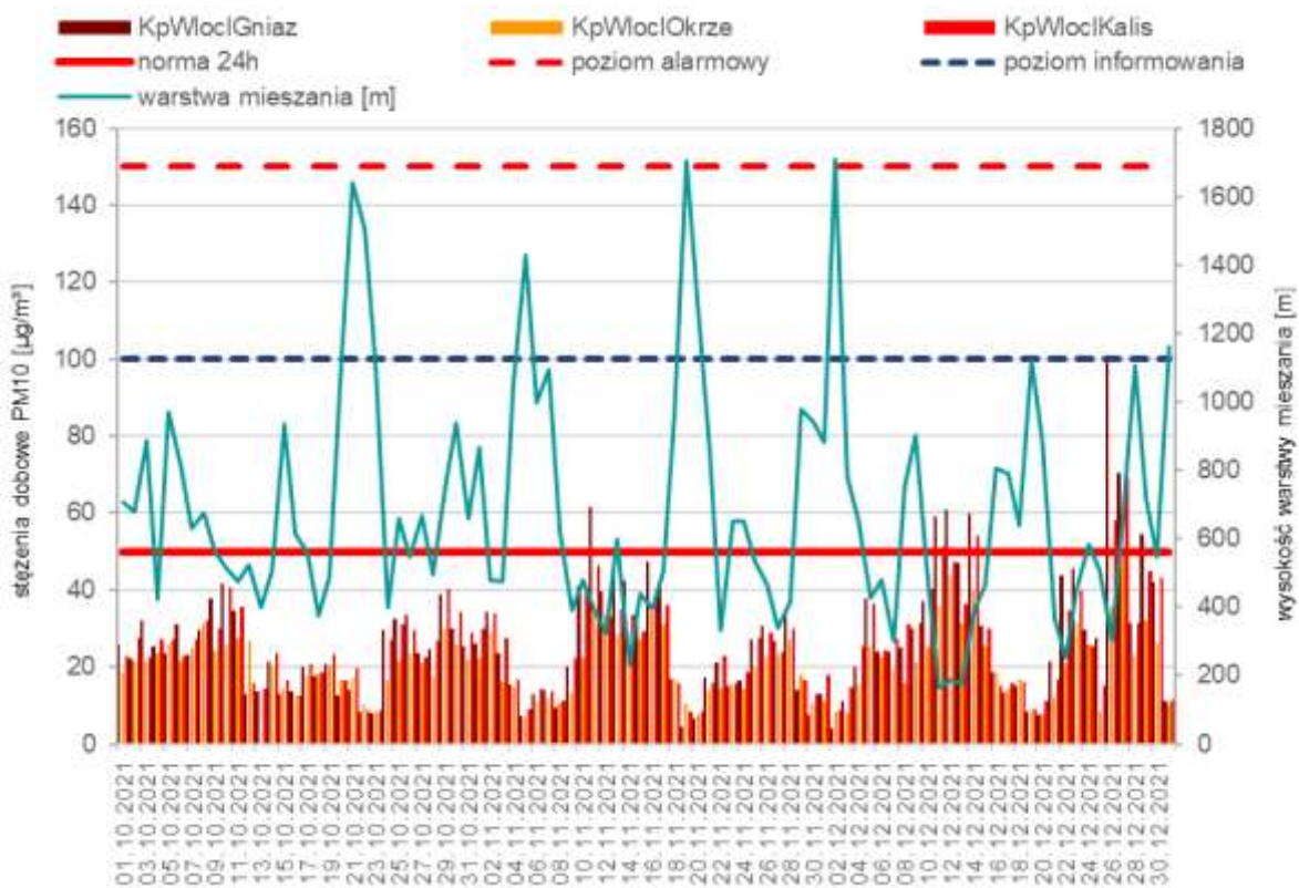
Rysunek 12. Porównanie przebiegu zmienności stężeń 24-godz. PM10 w IV kwartale 2021 r. we Włocławku z wysokością warstwy mieszanicy 53
