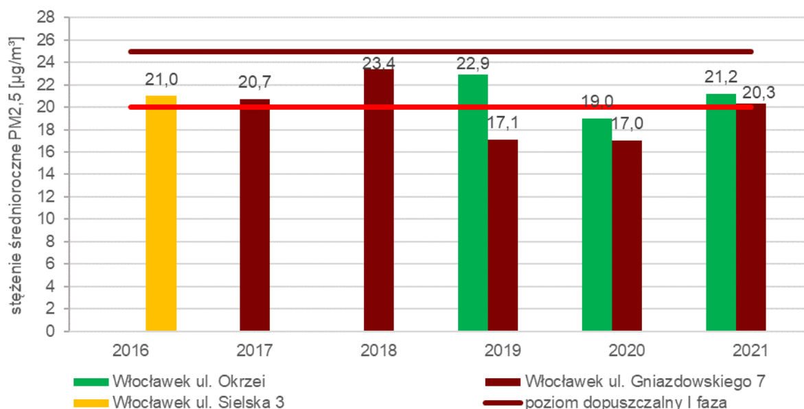
Rysunek 13. Stężenie średnioroczne pyłu zawieszonego PM 2,5 w latach 2016-2021 w strefie miasto Włocławek 55
