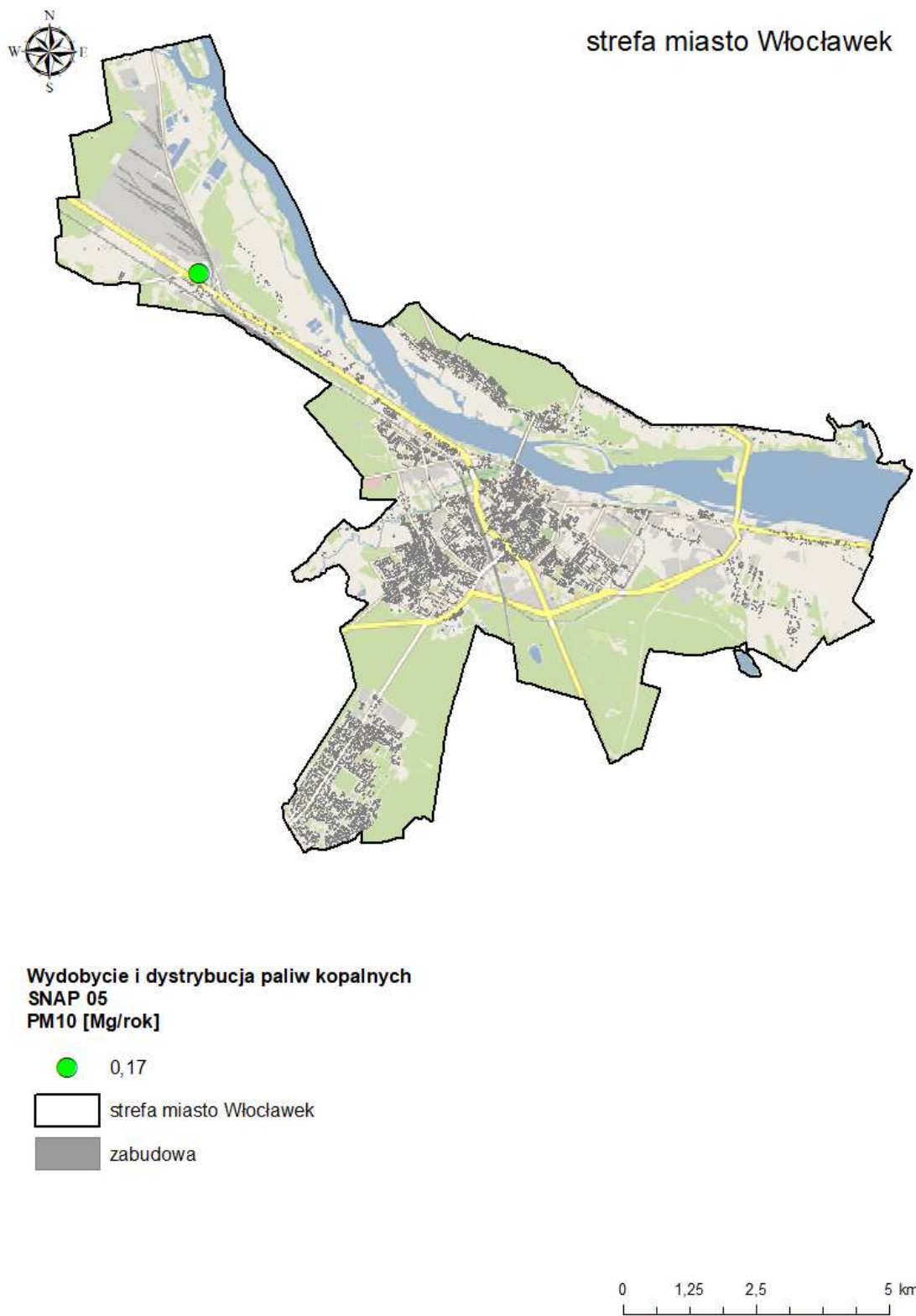
Rysunek 27. Emisja pyłu zawieszonego PM10 z wydobywania i dystrybucji paliw kopalnych (SNAP 05) 105
