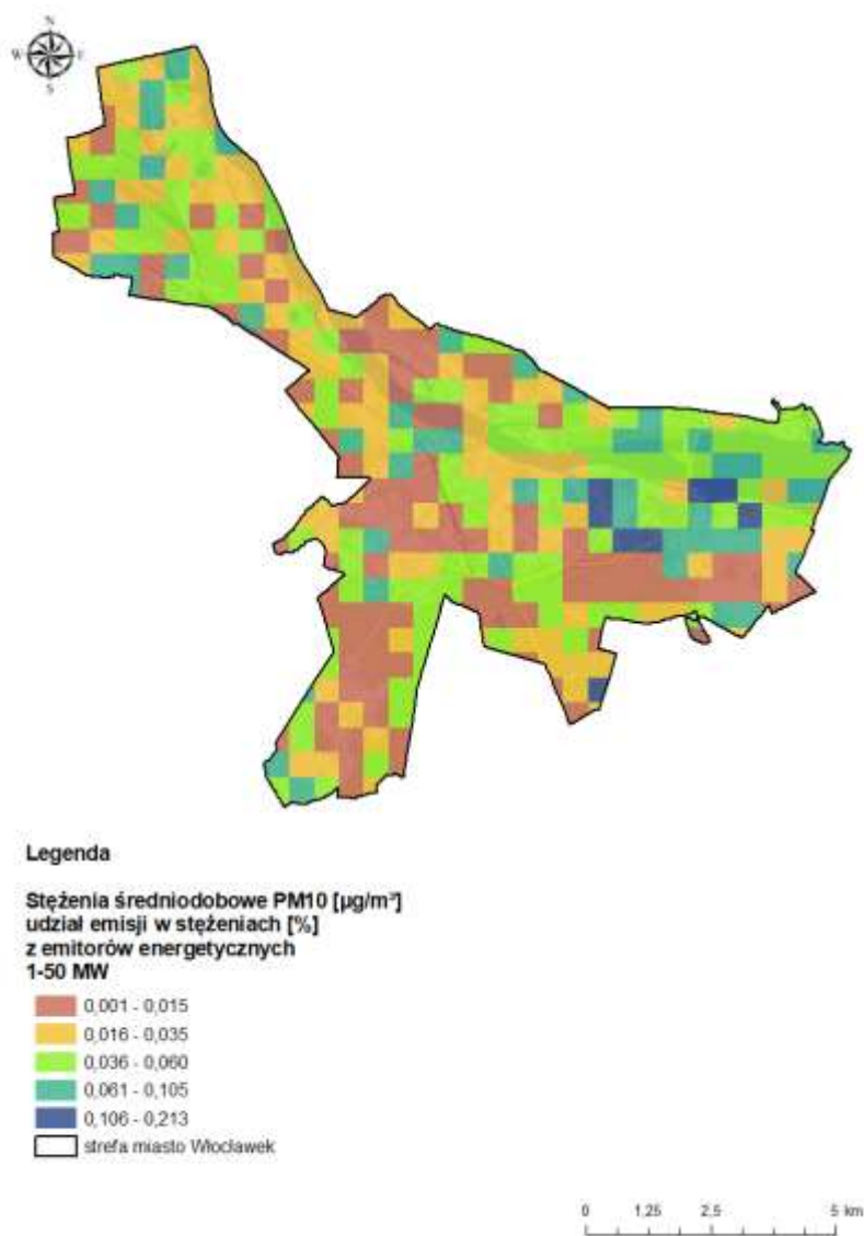
Rysunek 18. Udział [%] emisji ze źródeł o mocy 1-50 MW w strefie miasto Włocławek w średniodobowych stężeniach pyłu zawieszonoego PM10 (36 max) w 2021 r. 67
