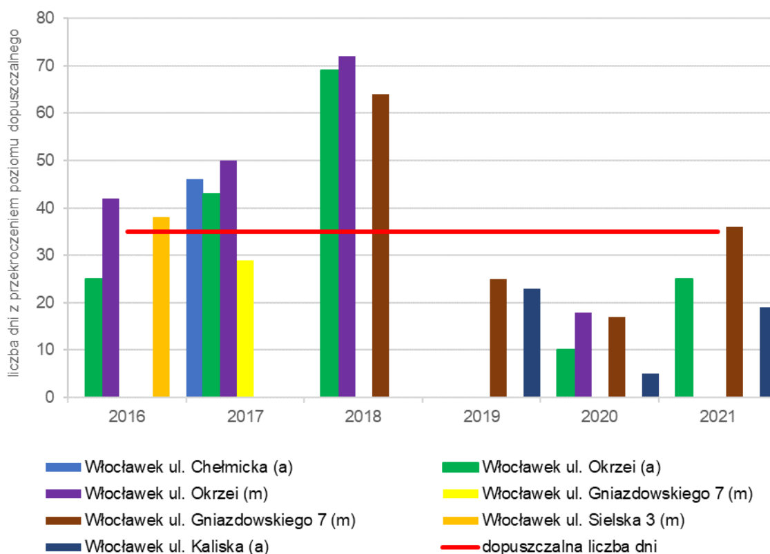
Rysunek 6. Liczba dni z przekroczeniem dopuszczalnego stężenia 24 godz. pyłu zawieszzonego PM10 w strefie miasto Włocławek w latach 2016-2021 44
