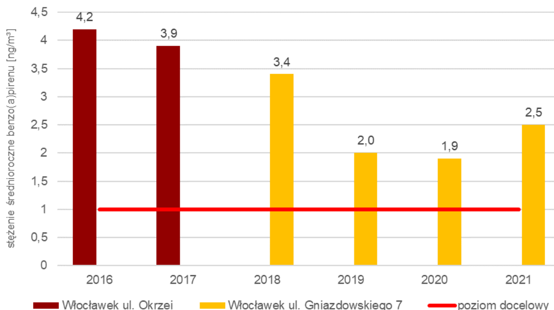
Rysunek 14. Stężenie średnioroczne benzo(a)pirenu w latach 2016-2021 w strefie miasto Włocławek 58
