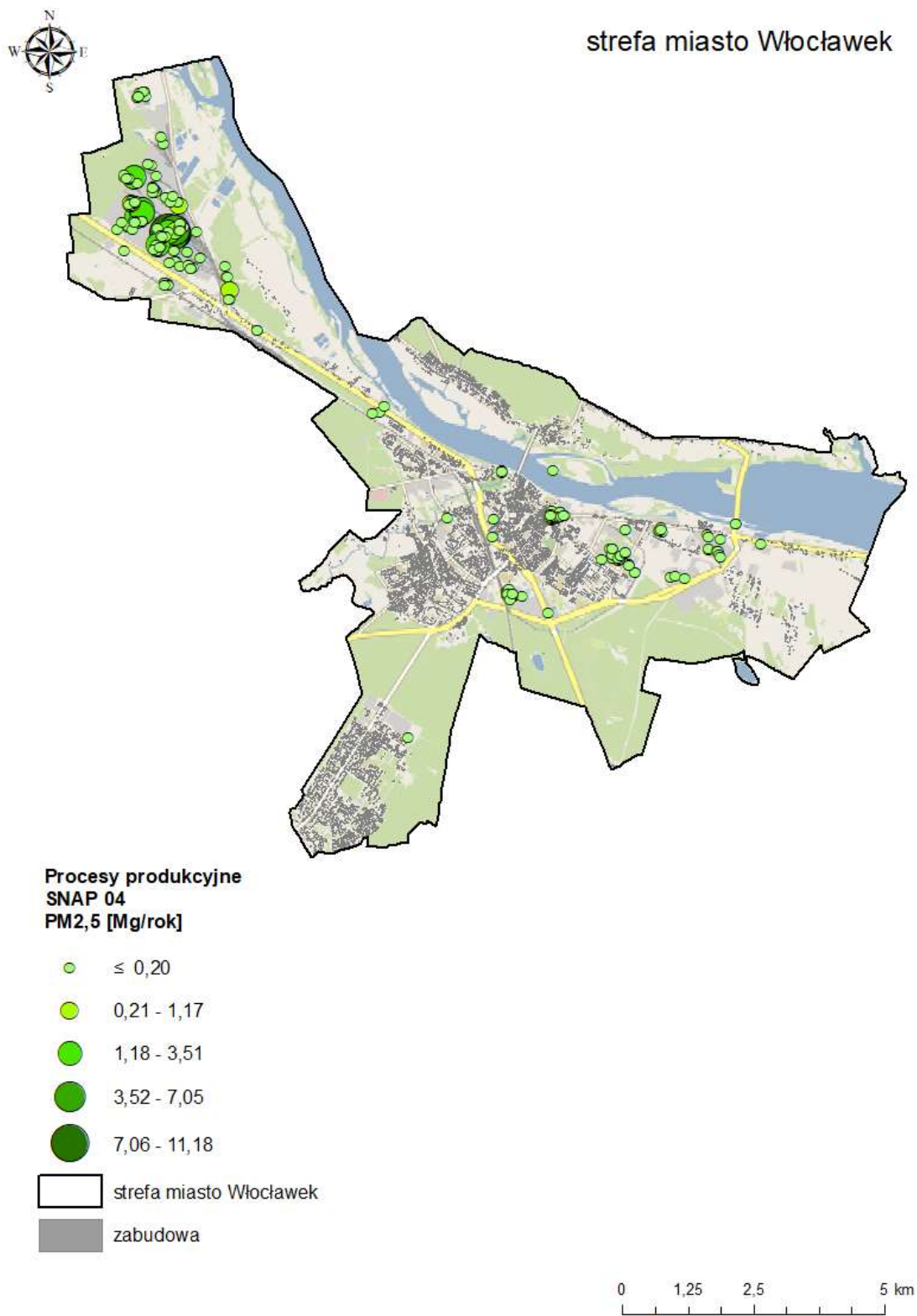
Rysunek 36. Emisja pyłu zawieszonego PM 2,5 z procesów produkcyjnych (SNAP 04) 114
