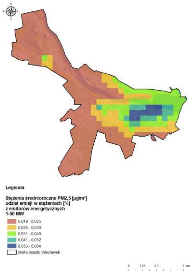
Rysunek 20. Udział [%] emisji ze źródeł o mocy 1-50 MW w strefie miasto Włocławek w średniorocznych stężeniach pyłu zawieszonego PM 2,5 w 2021 r. 69
