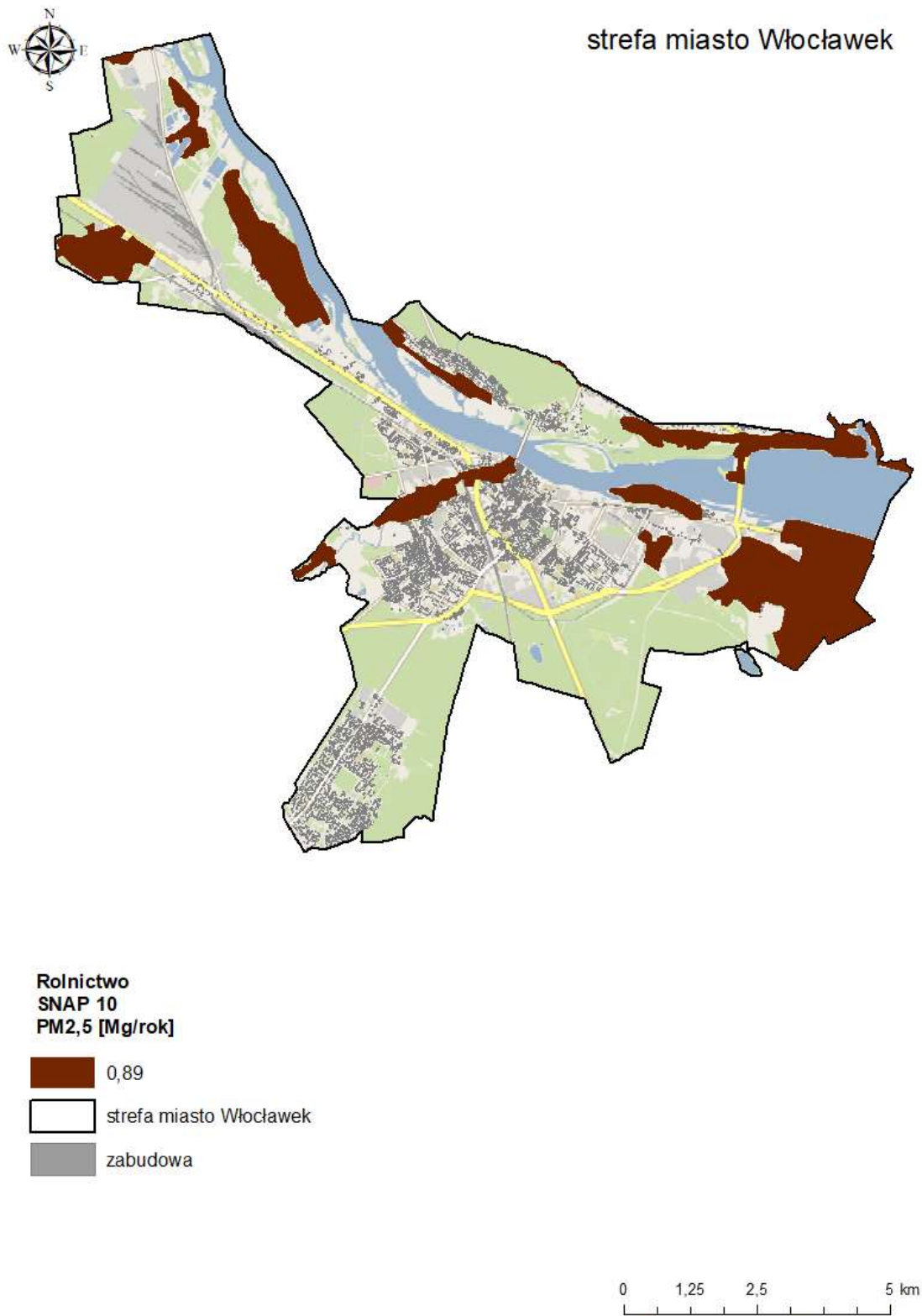
Rysunek 41. Emisja pyłu zawieszonego PM2,5 z rolnictwa (SNAP 10) 119
