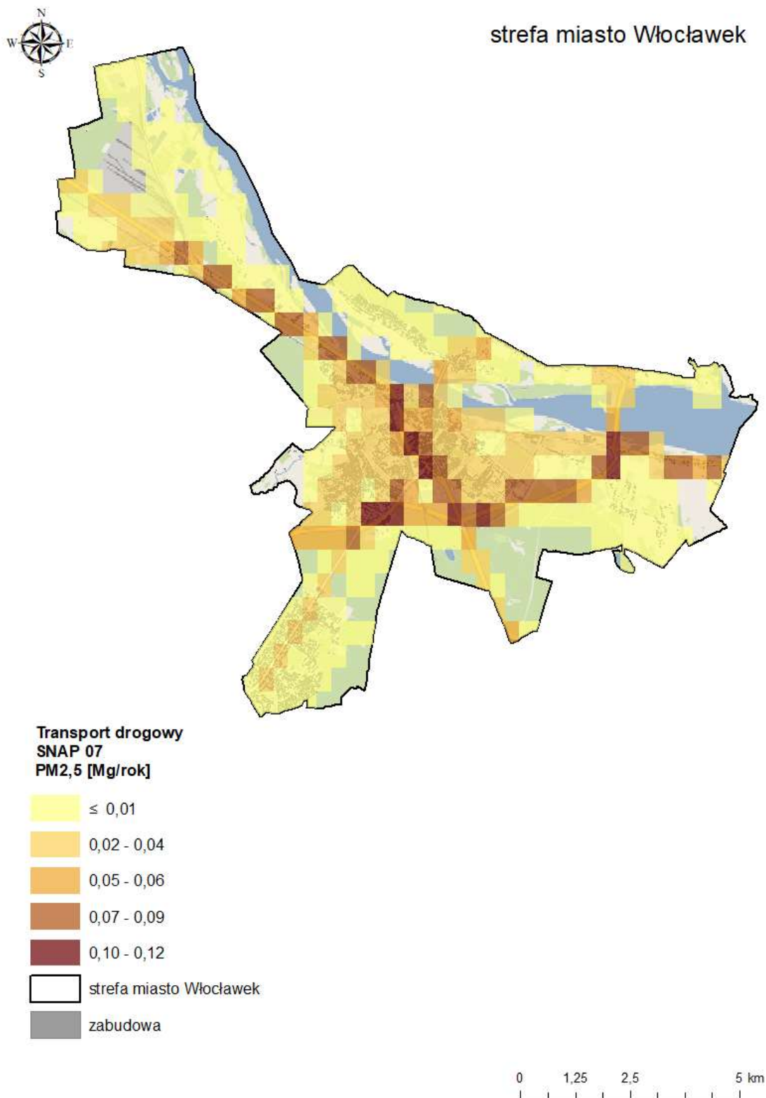
Rysunek 38. Emisja pyłu zawieszonego PM2,5 z transportu drogowego (SNAP 07) 116
