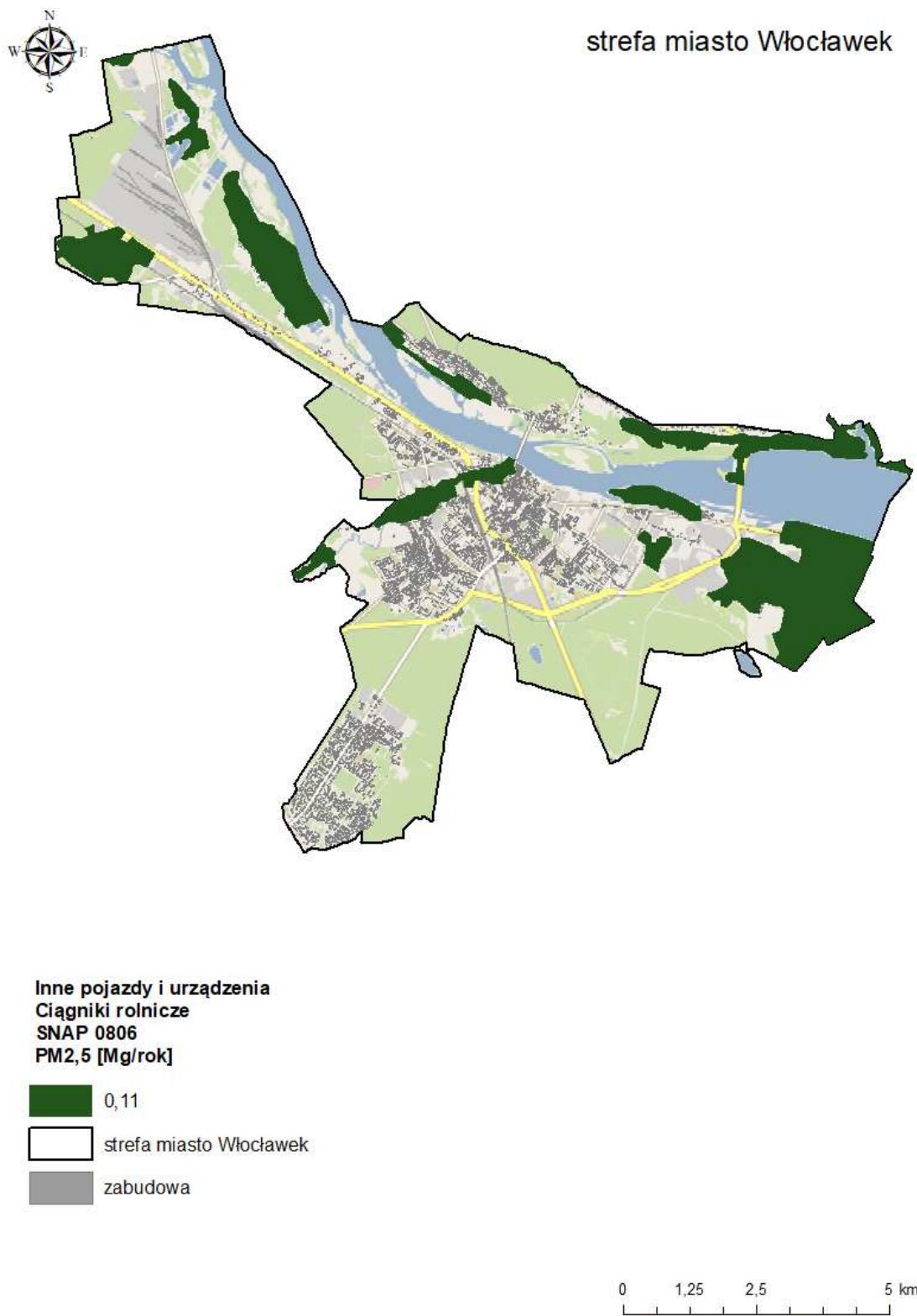
Rysunek 40. Emisja pyłu zawieszonoego PM 2,5 z innych pojazdów i urządzeń - ciągników rolniczych (SNAP 0806) 118
