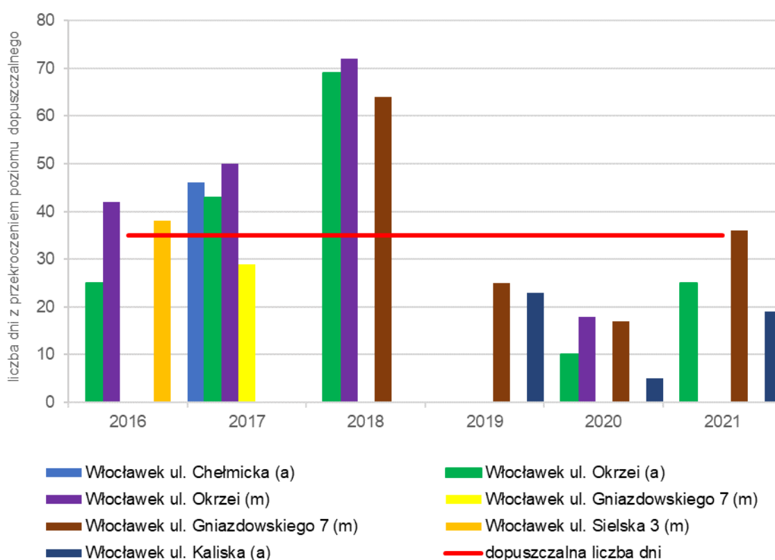
Rysunek 6. Liczba dni z przekroczeniem dopuszczalnego stężenia 24 godz. pyłu zawieszony PM10 w strefie miasto Włocławek w latach 2016-2021 44
