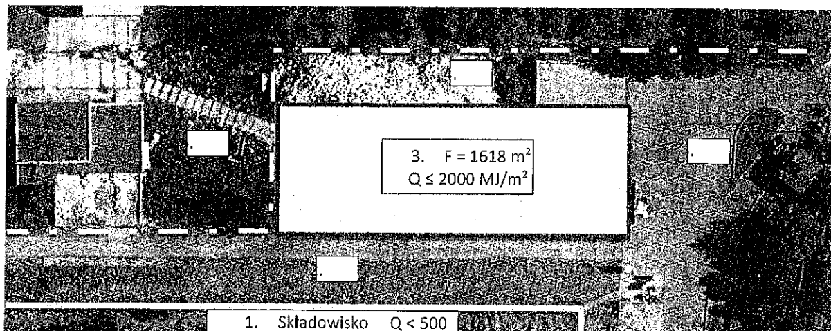
Rysunek 2. Dopuszczalny sposób magazynowania odpadów w przypadku braku ściany oddzielenia przeciwpożarowego od granicy działki.
