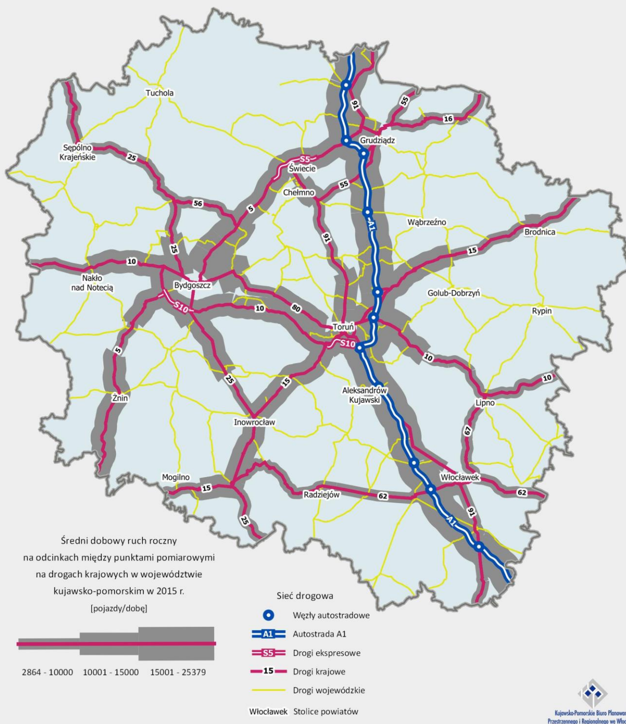
Rysunek 21. Średni dobowy ruch roczny na odcinkach między punktami pomiarowymi na drogach krajowych przebiegających przez obszar województwa kujawsko-pomorskiego w 2015 r.
