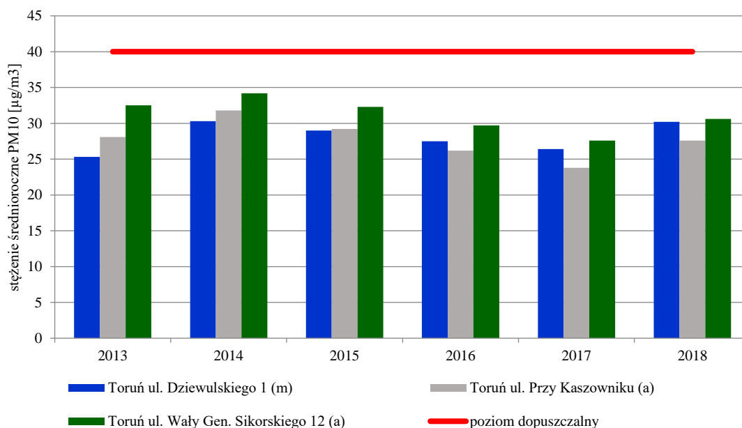
Rysunek 5. Stężenie średnioroczne PM10 w strefie miasto Toruń 41
