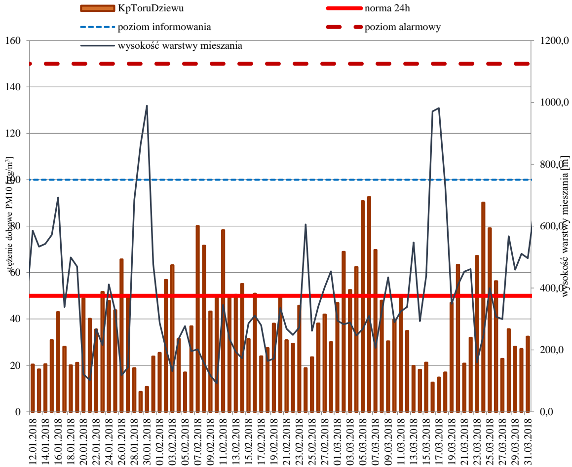
Rysunek 8. Porównanie przebiegu zmienności stężeń 24-godz. PM10 w I kwartale 2018 r. w Toruniu z wysokością warstwy mieszanania 48
