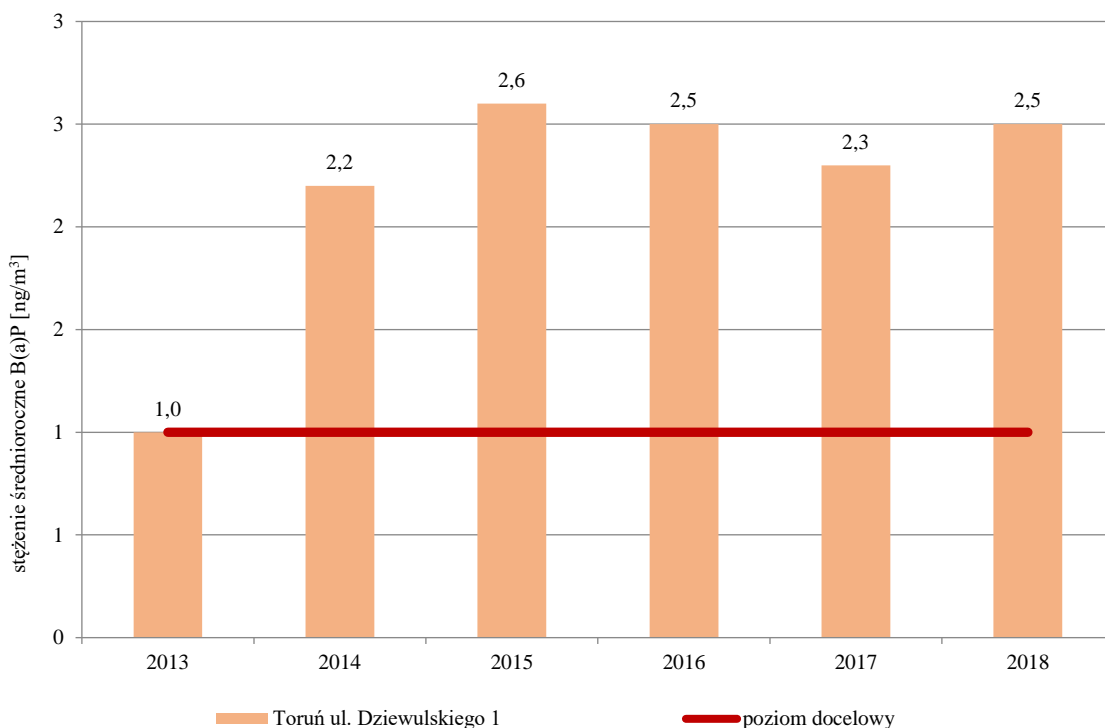
Rysunek 12. Stężenie średnioroczne benzo(a)pirenu w strefie miasto Toruń 52
