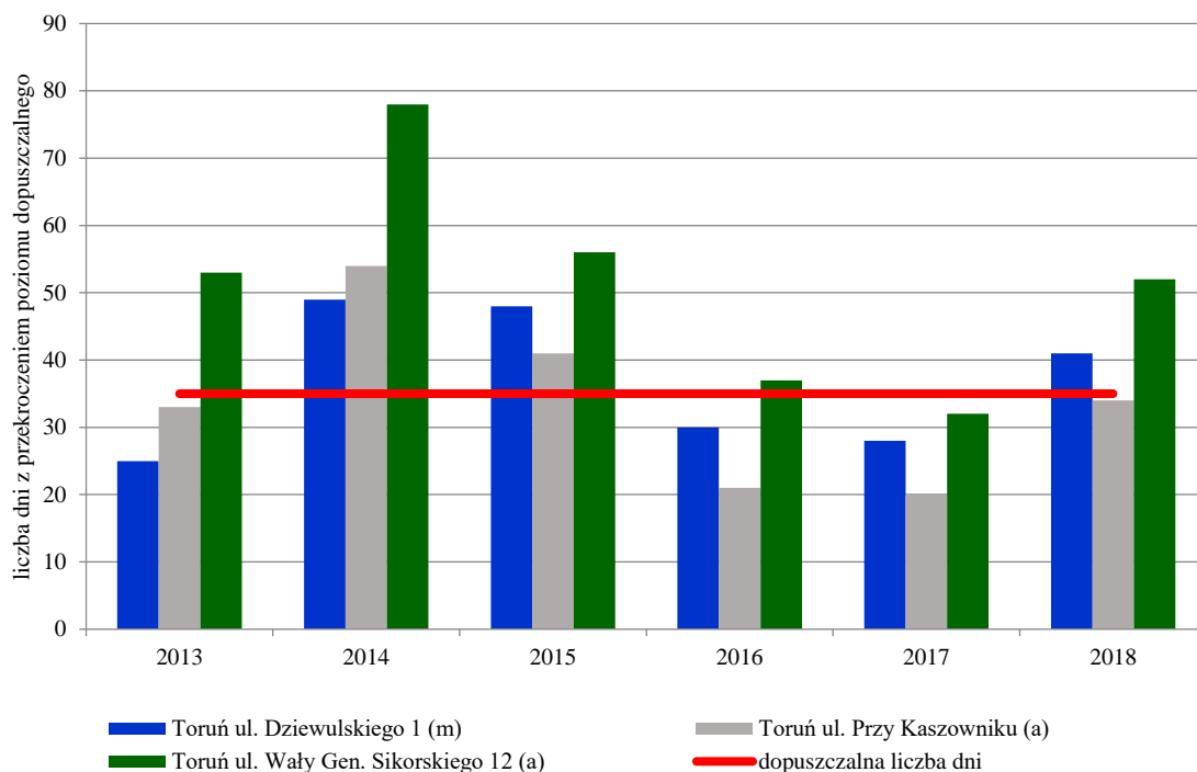
Rysunek 4. Liczba dni z przekroczeniem dopuszczalnego stężenia 24-godz. PM10 w strefie miasto Toruń w latach 2013-2018 40
