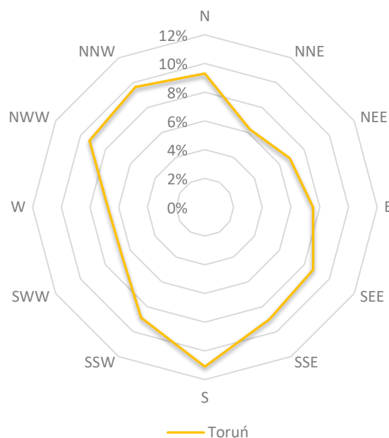
Rysunek 2. Róża wiatrów dla miasto Toruń 30
