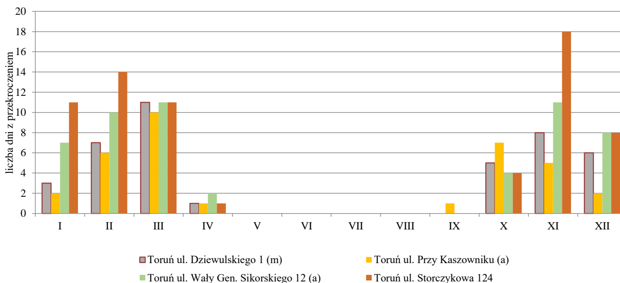
Rysunek 3. Liczba dni z przekroczeniem dopuszczalnego stężenia 24-godz. PM10 w 2018 roku. 39
