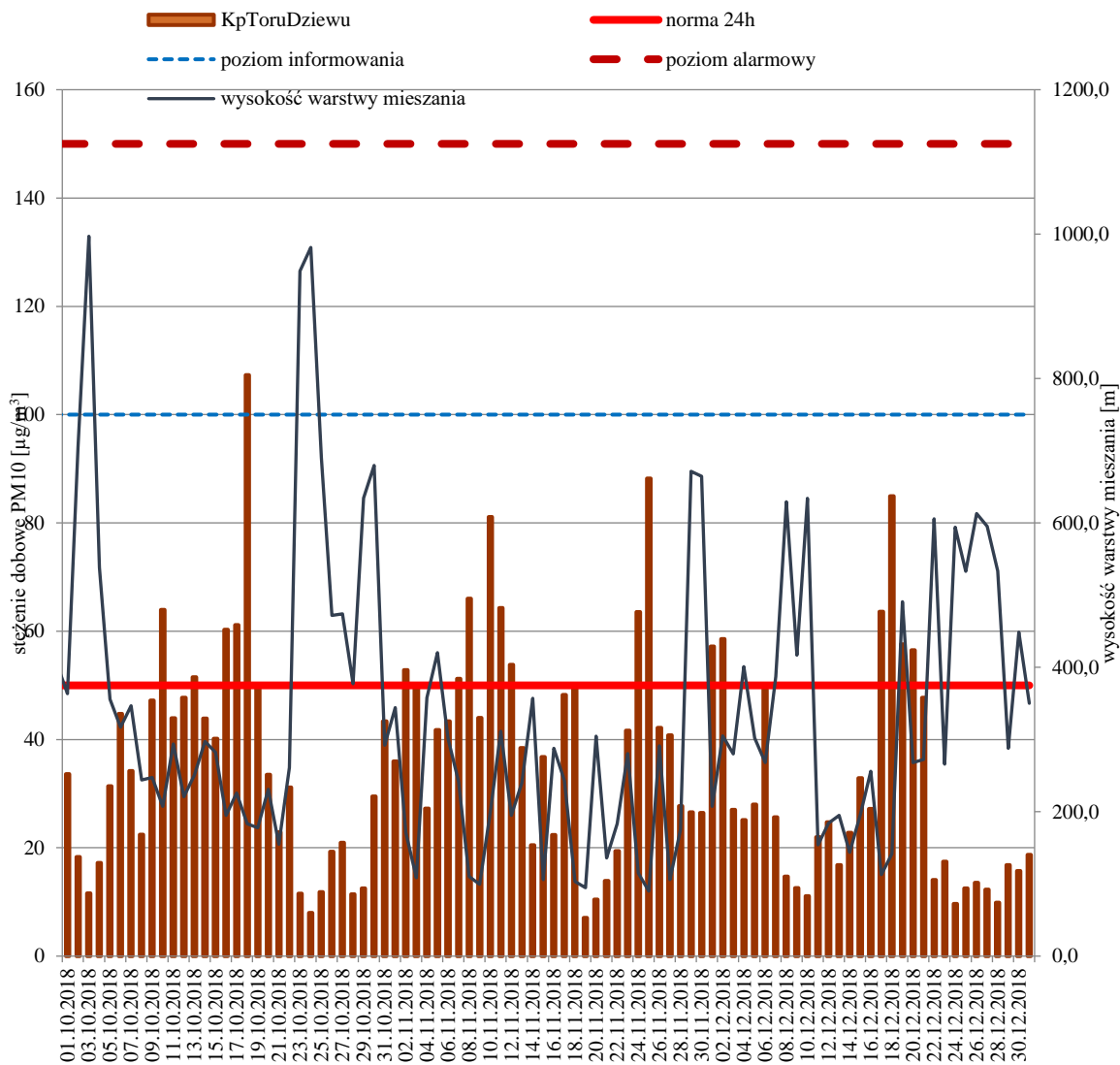
Rysunek 9. Porównanie przebiegu zmienności stężeń 24-godz. PM10 w IV kwartale 2018 r. w Toruniu z wysokością warstwy mieszaną 49
