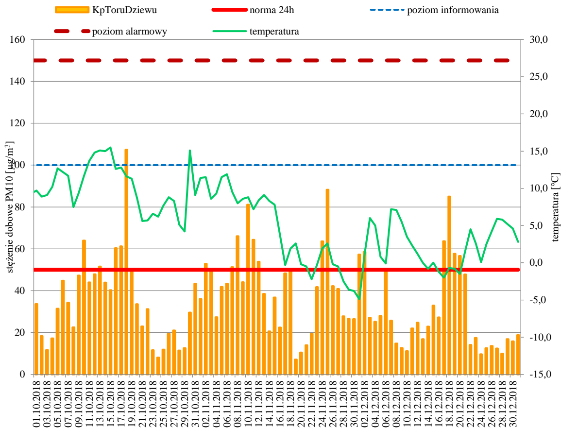
Rysunek 11. Porównanie przebiegu zmienności stężeń 24-godz. PM10 w IV kwartale 2018 r. w Toruniu z temperaturą 51
