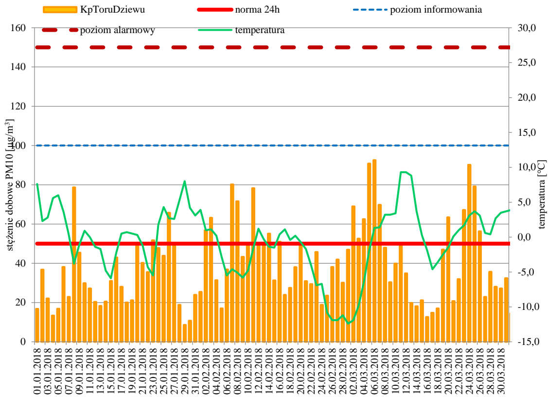
Rysunek 10. Porównanie przebiegu zmienności stężeń 24-godzinnych PM10 w I kwartale 2018 r. w Toruniu z temperaturą 50
