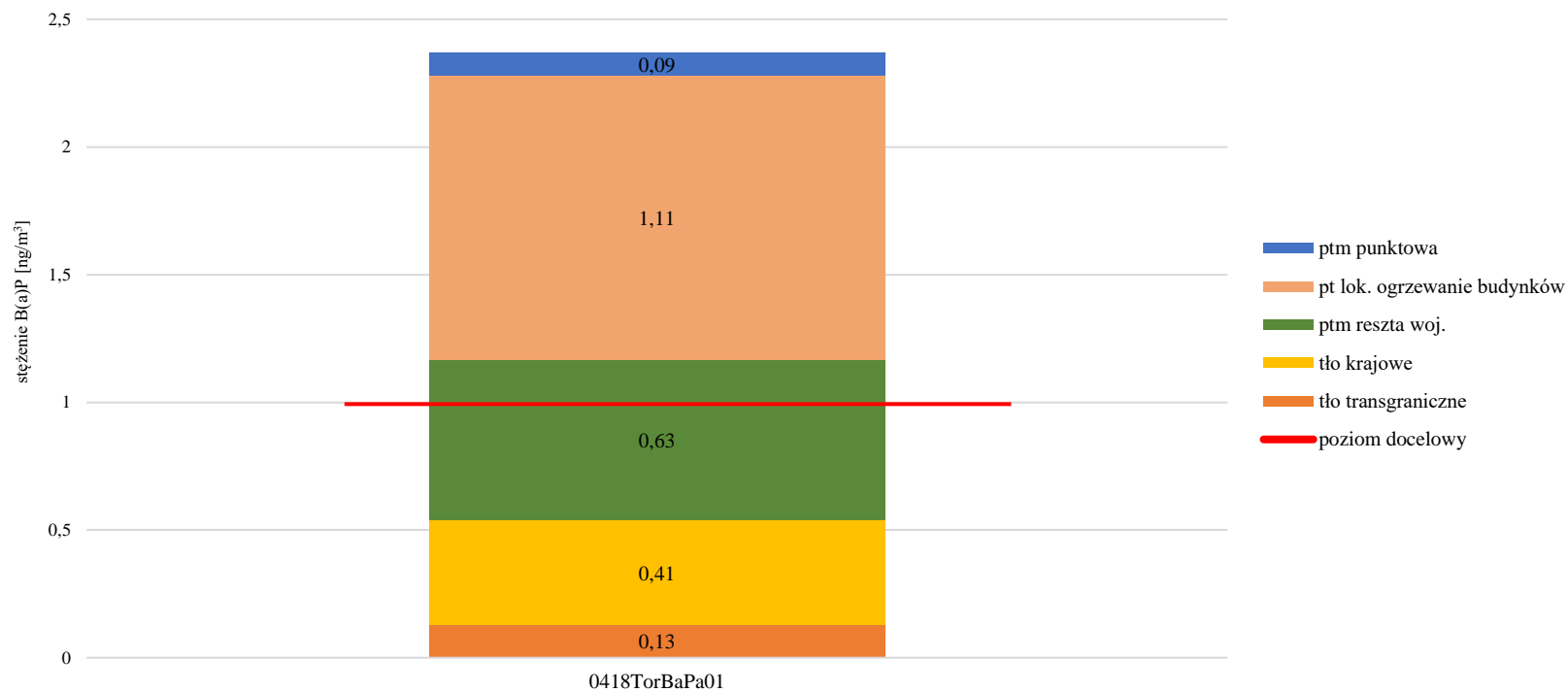
Rysunek 16. Obszar przekroczeń poziomu docelowego benzo(a)pirenu w Toruniu 63
