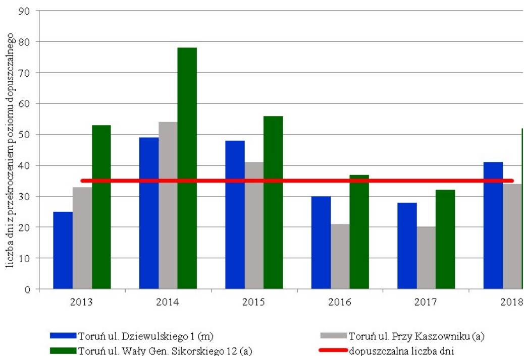
Rysunek 4. Liczba dni z przekroczeniem dopuszczalnego stężenia 24-godz. PM10 w strefie miasto Toruń w latach 2013-2018 39
