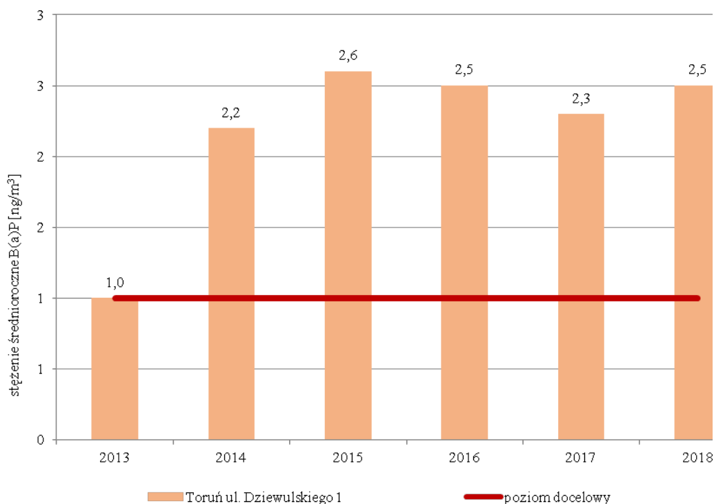
Rysunek 12. Stężenie średnioroczne benzo(a)pirenu w strefie miasto Toruń 48
