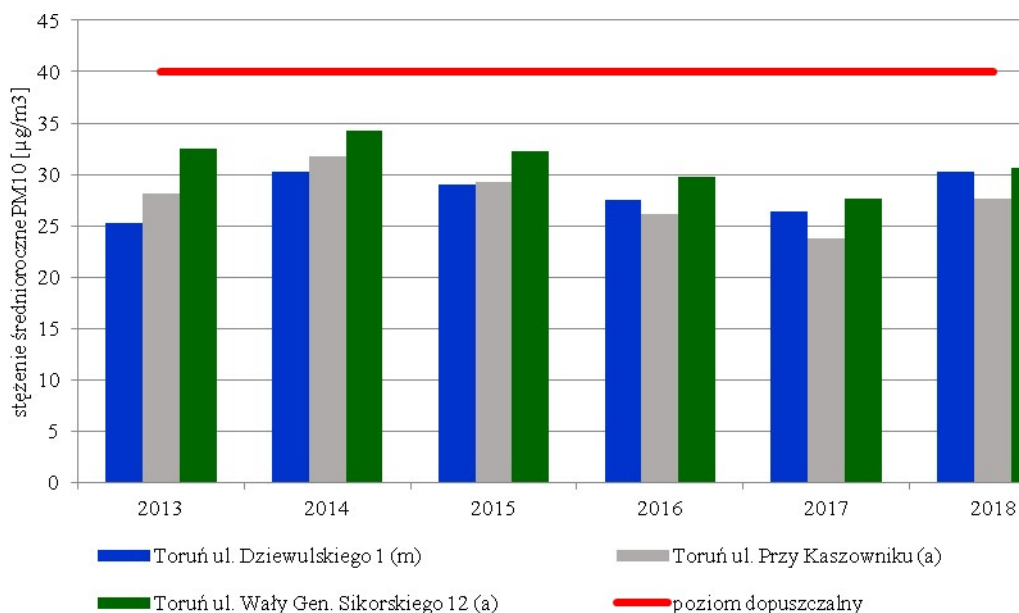
Rysunek 5. Stężenie średnioroczne PM10 w strefie miasto Toruń 40
