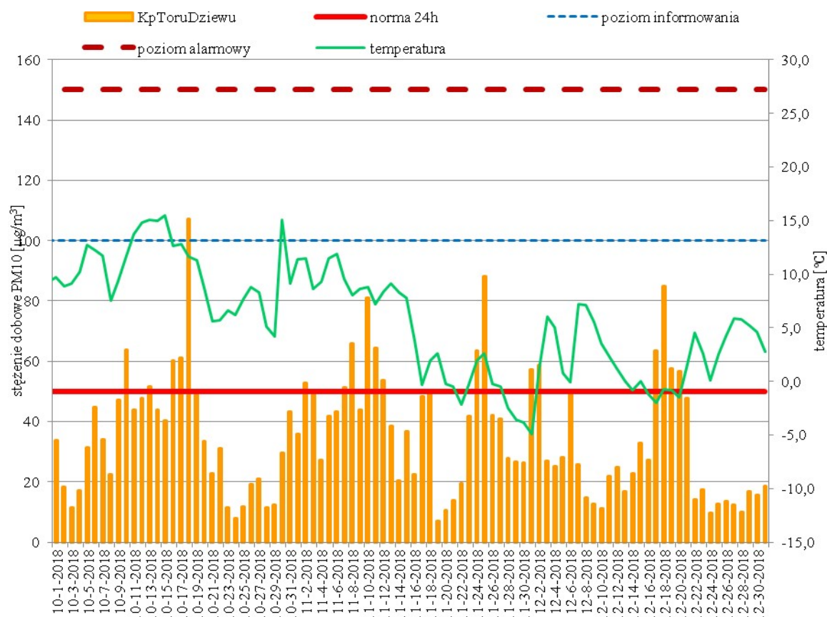
Rysunek 11. Porównanie przebiegu zmienności stężeń 24-godz. PM10 w IV kwartale 2018 r. w Toruniu z temperaturą 47
