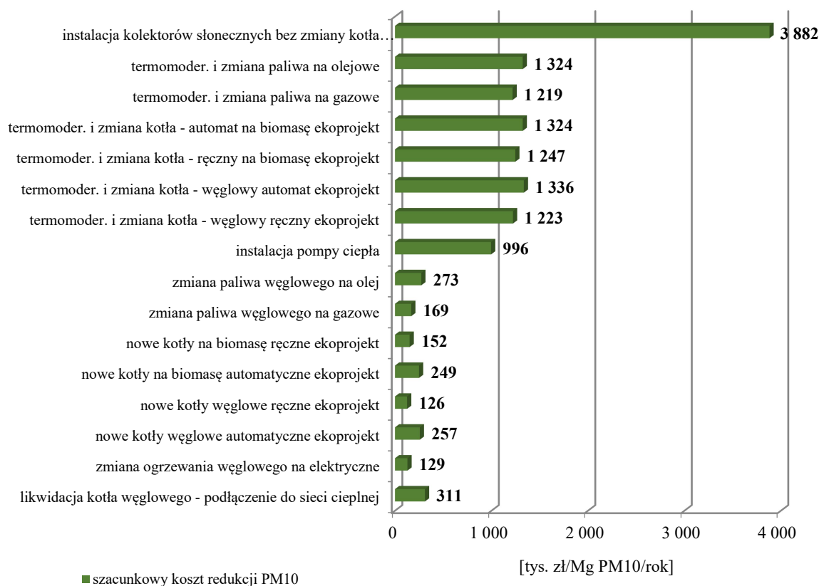
Rysunek 33. Porównanie szacunkowych, średnich wskaźników kosztów redukcji pyłu zawieszonoego PM10 z indywidualnych systemów grzewczych 117
