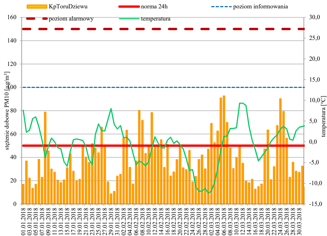
Rysunek 10. Porównanie przebiegu zmienności stężeń 24-godz. PM10 w I kwartale 2018 r. w Toruniu z temperaturą 46
