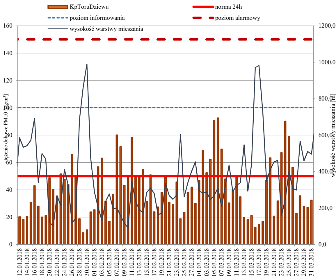
Rysunek 8. Porównanie przebiegu zmienności stężeń 24-godz. PM10 w I kwartale 2018 r. w Toruniu z wysokością warstwy mieszania 44
