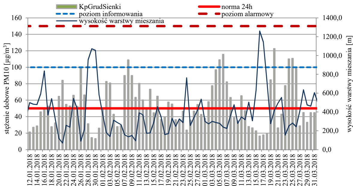
Rysunek 9. Porównanie przebiegu zmienności stężeń 24-godz. PM10 w I kwartale 2018 r. w Grudziądzu z wysokością warstwy mieszanania 49
