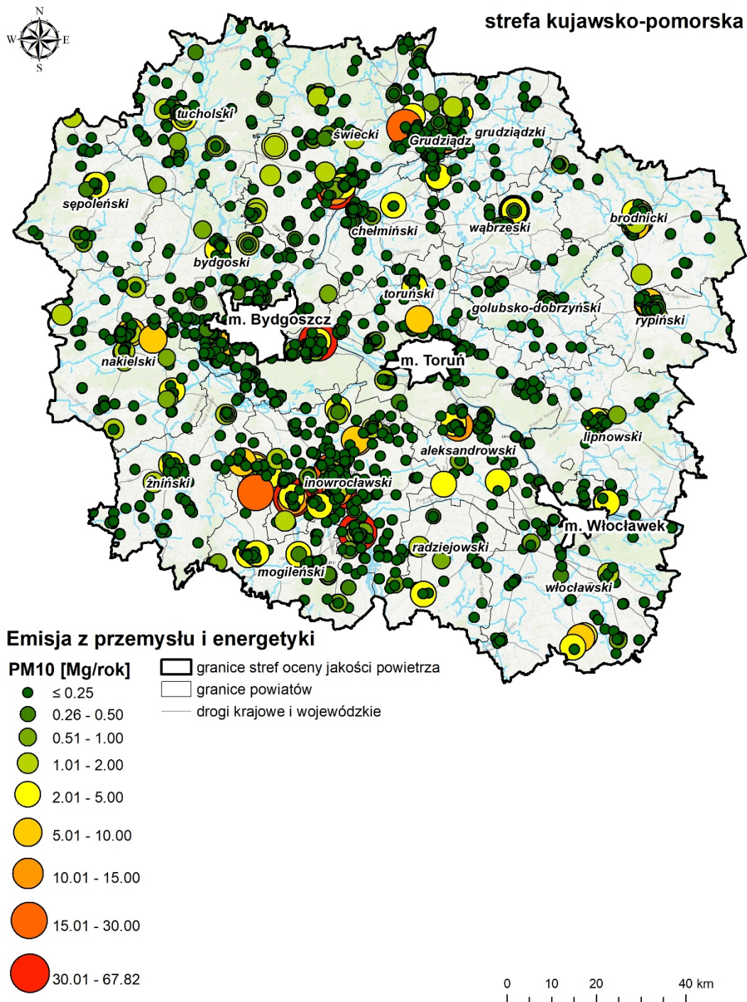
Rysunek 20. Emisja pyłu zawieszzonego PM10 ze źródeł przemysłowych i energetycznych 79
