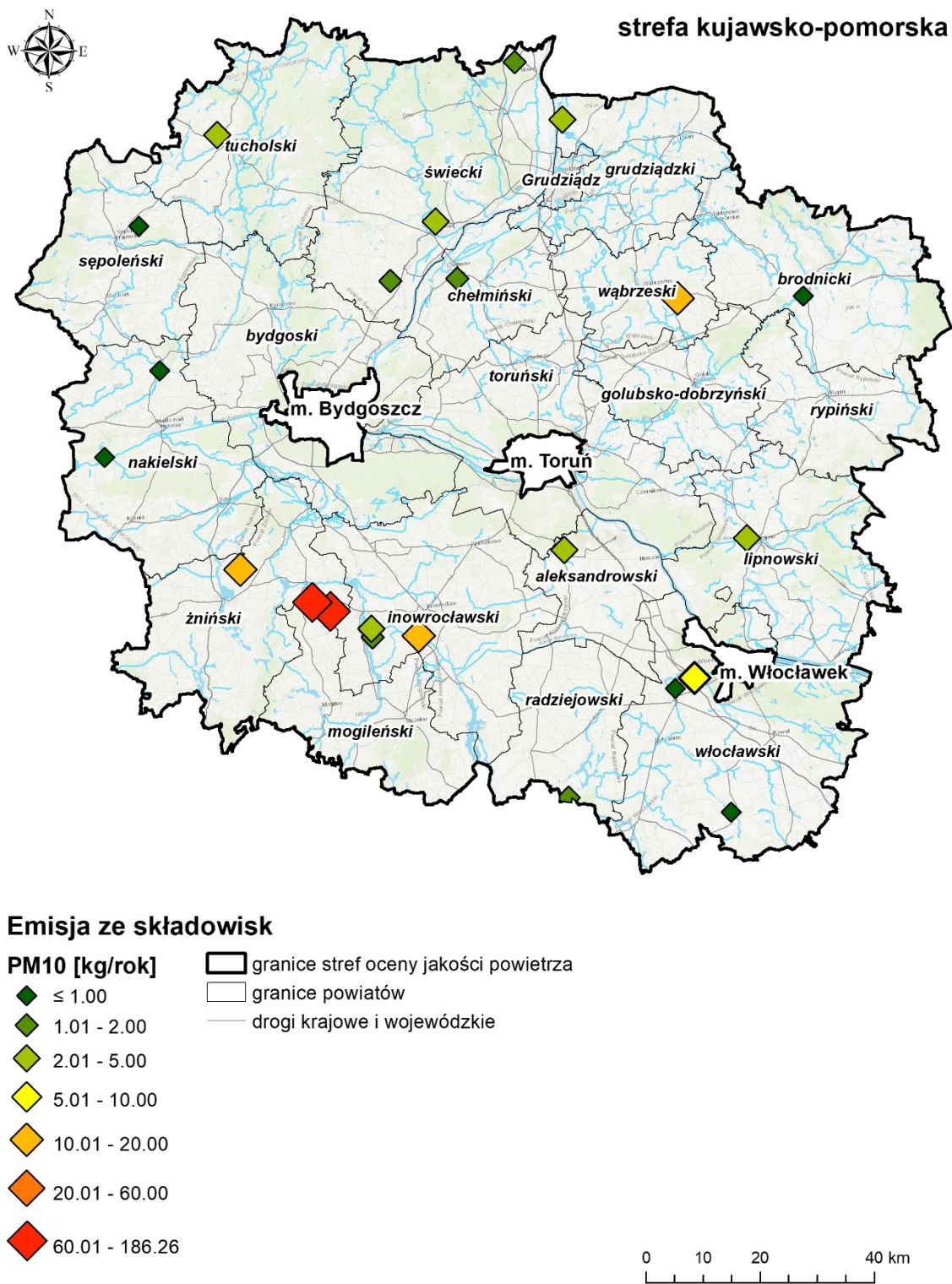
Rysunek 25. Emisja pyłu zawieszonego PM10 ze składowisk odpadów 84
