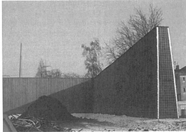
Rysunek 36. Przykładowy ekran akustyczny – ziemny ekran akustyczny z konstrukcją stalową. [Źródło: Ecotec Polska]
