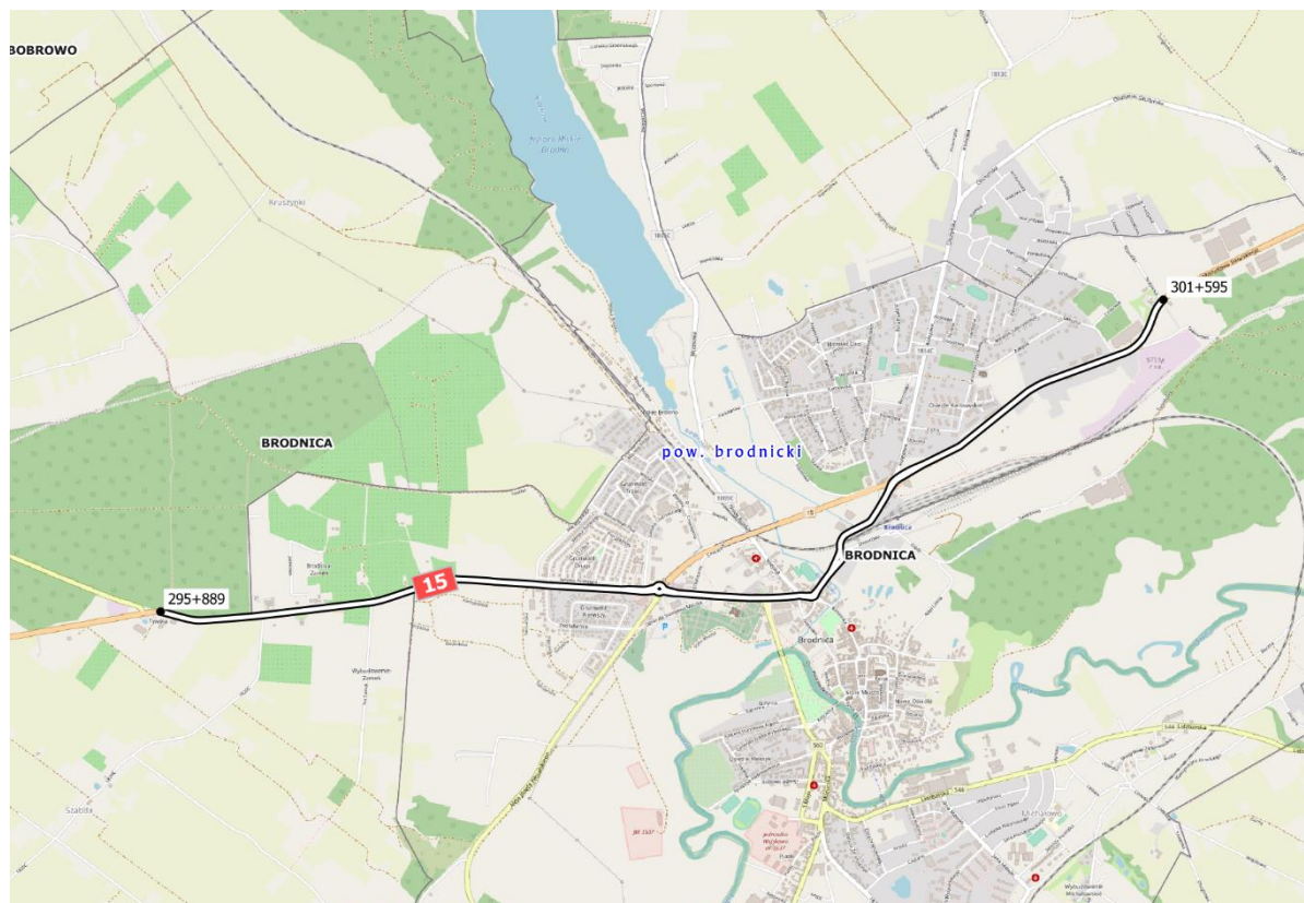
Rysunek 13. Lokalizacja pierwszego z analizowanych odcinków drogi krajowej nr 15 dla km 295+889 – 301+595 [Źródło: Opracowanie własne]
